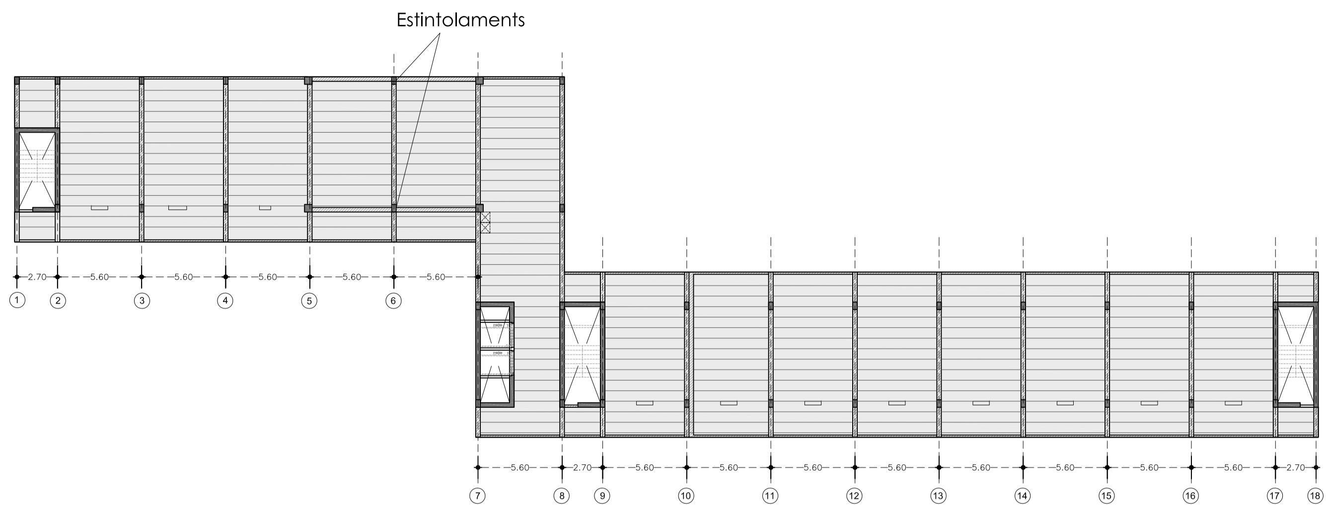
FORJAT NIVELL: +9.05
