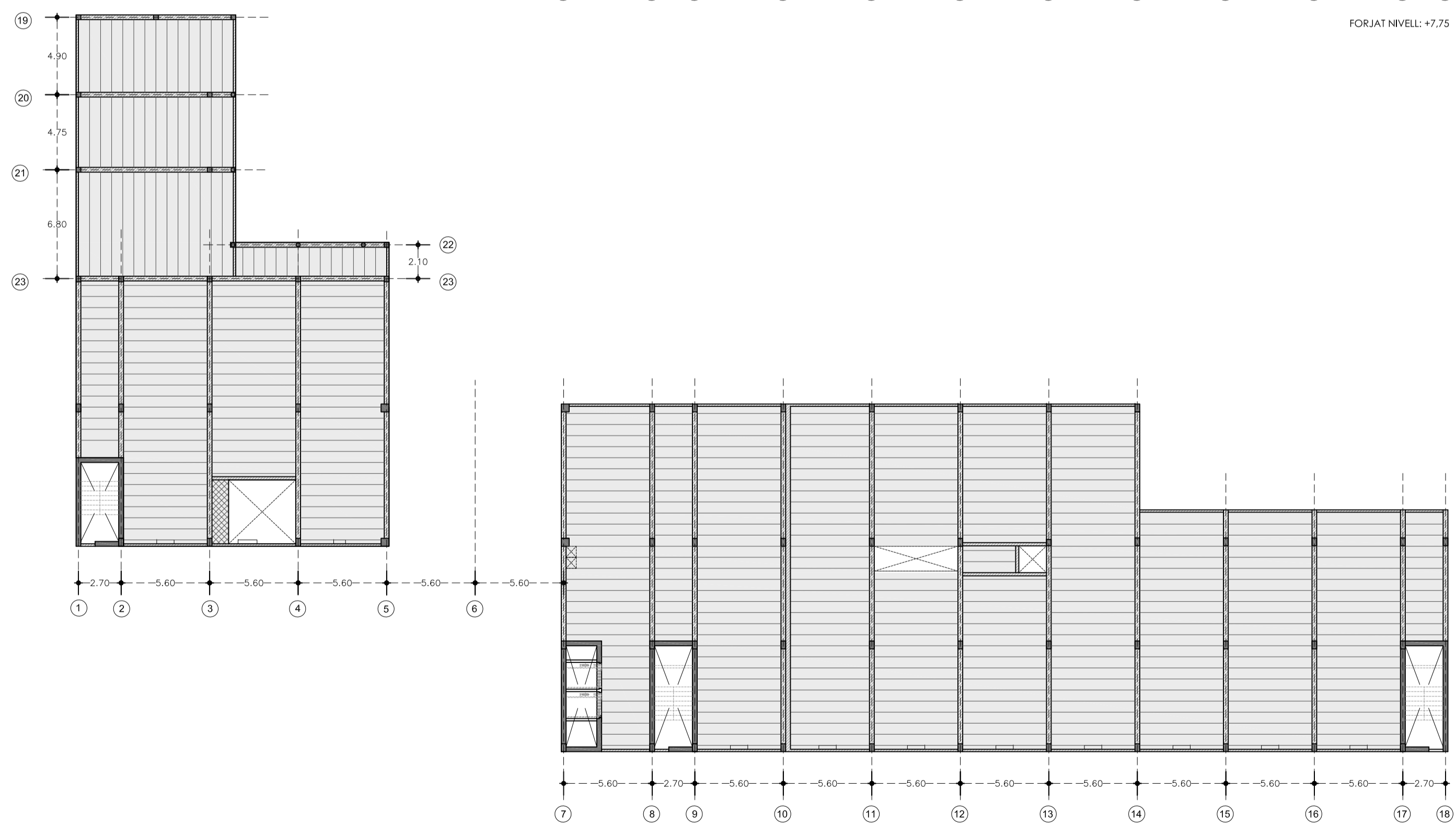
FORJAT NIVELL: +4.05
