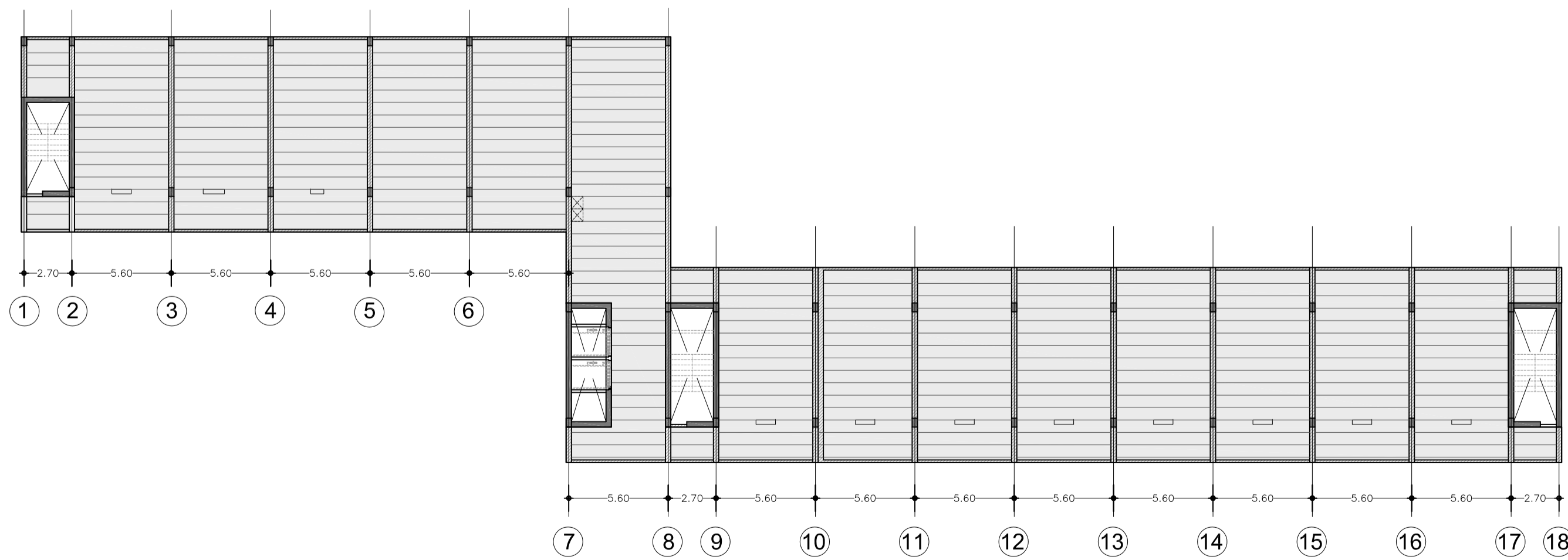
FORJAT NIVELL: +12.05/ +15.05/ +18.05
