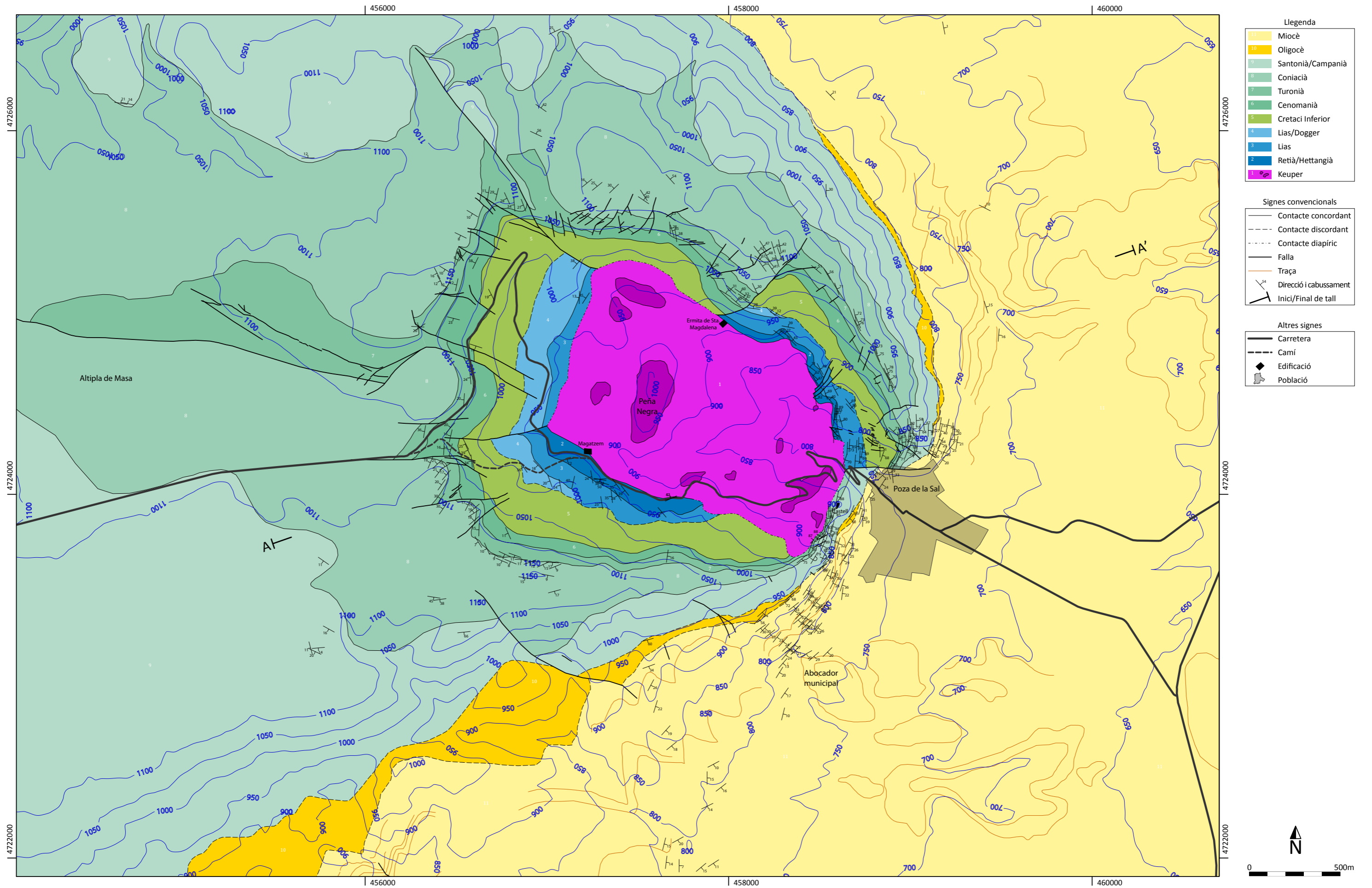
Figura 32. Cartografia geològica del diapir de Poza de la Sal
