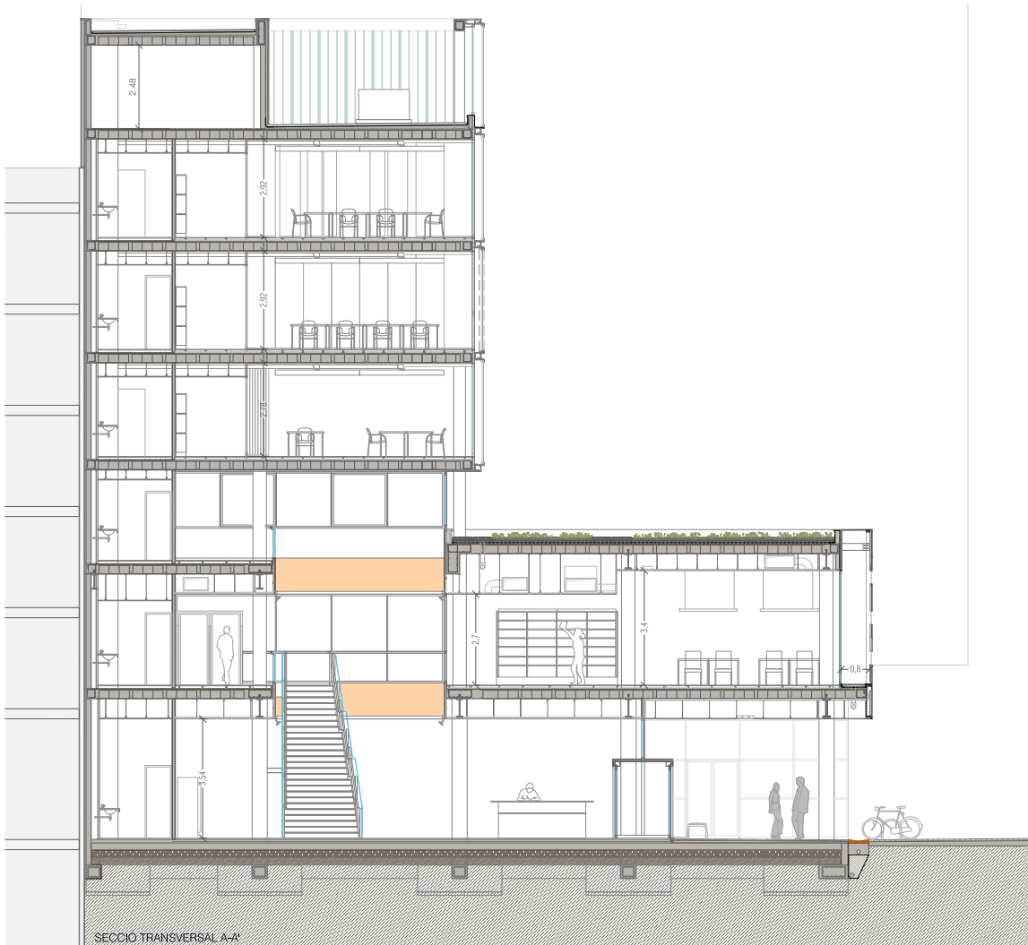
SECCIÓ TRANSVERSAL A-A'
