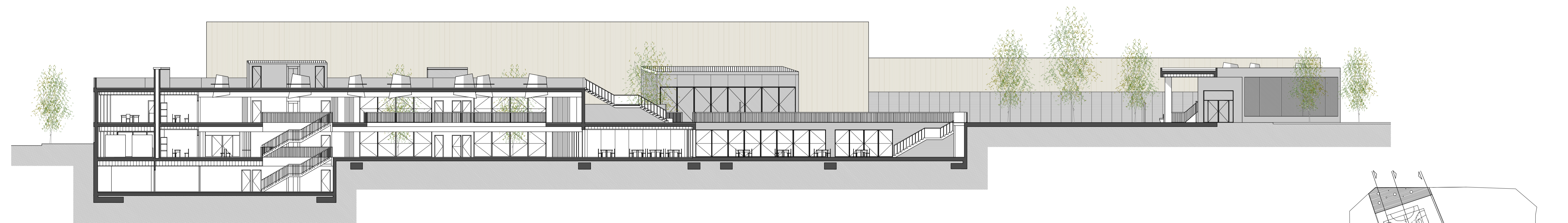
SECCIÓ LONGITUDINAL C-C' E:1/200
