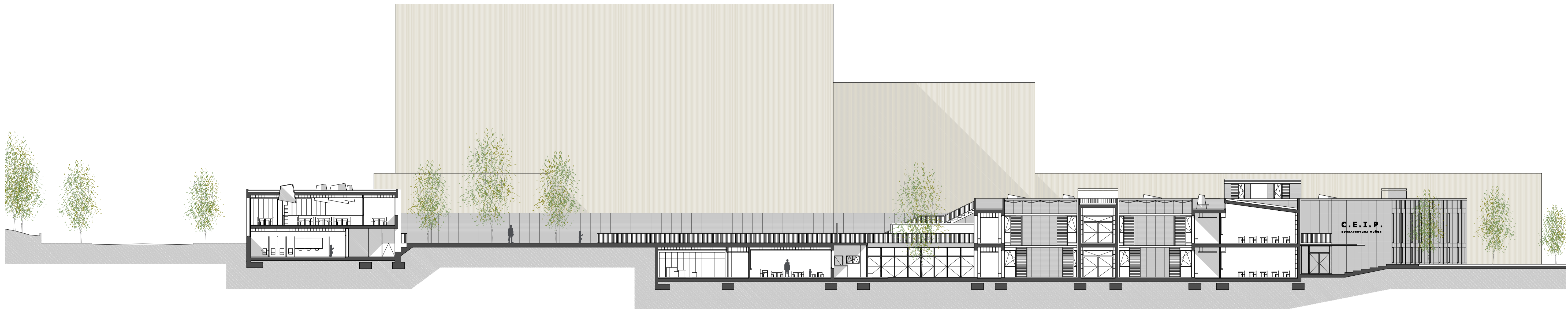
SECCIÓ LONGITUDINAL B-B' E:1/200
