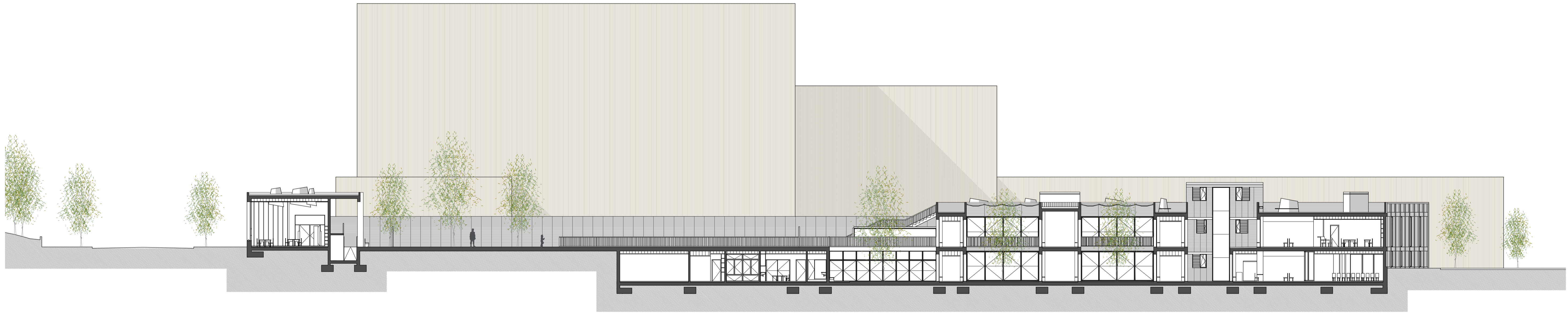
SECCIÓ LONGITUDINAL C-C' E:1/200
