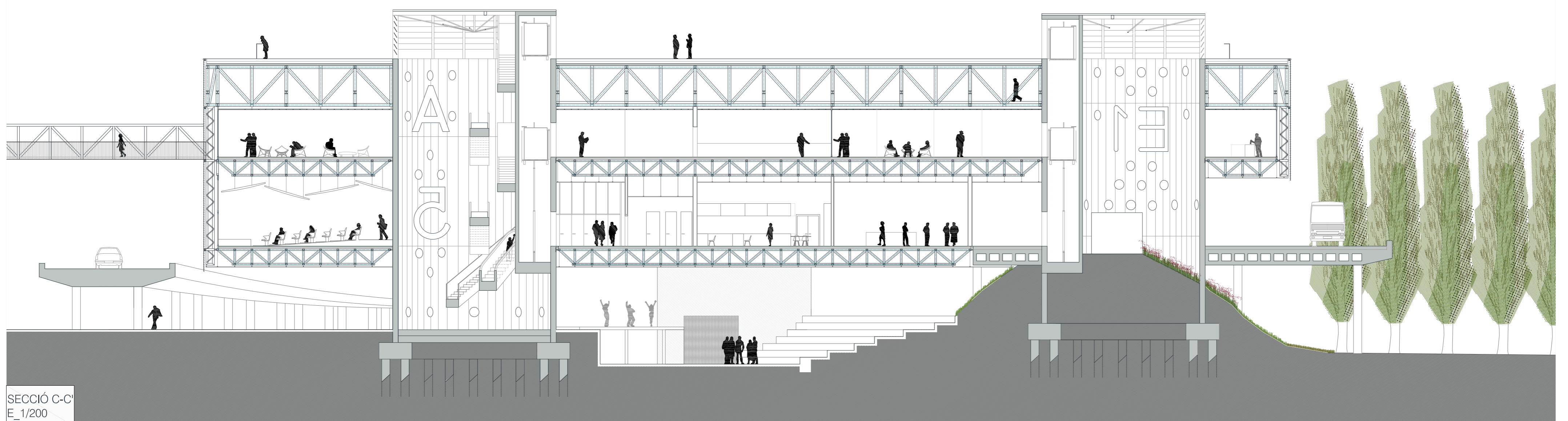
PLANTA NIVELL +67 E_1/200
