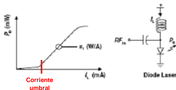
Figura 1.7. Curva característica y esquemático de un diodo láser.
