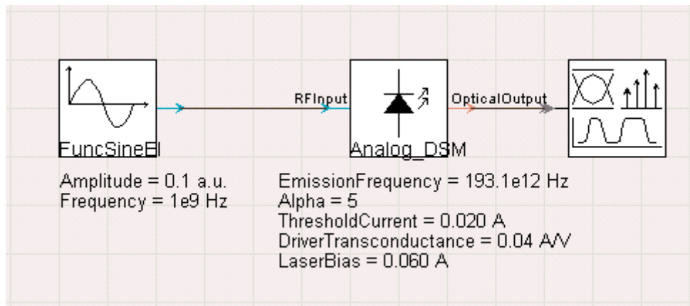
Figura 5.7. Esquema del circuito simulado en VPI
