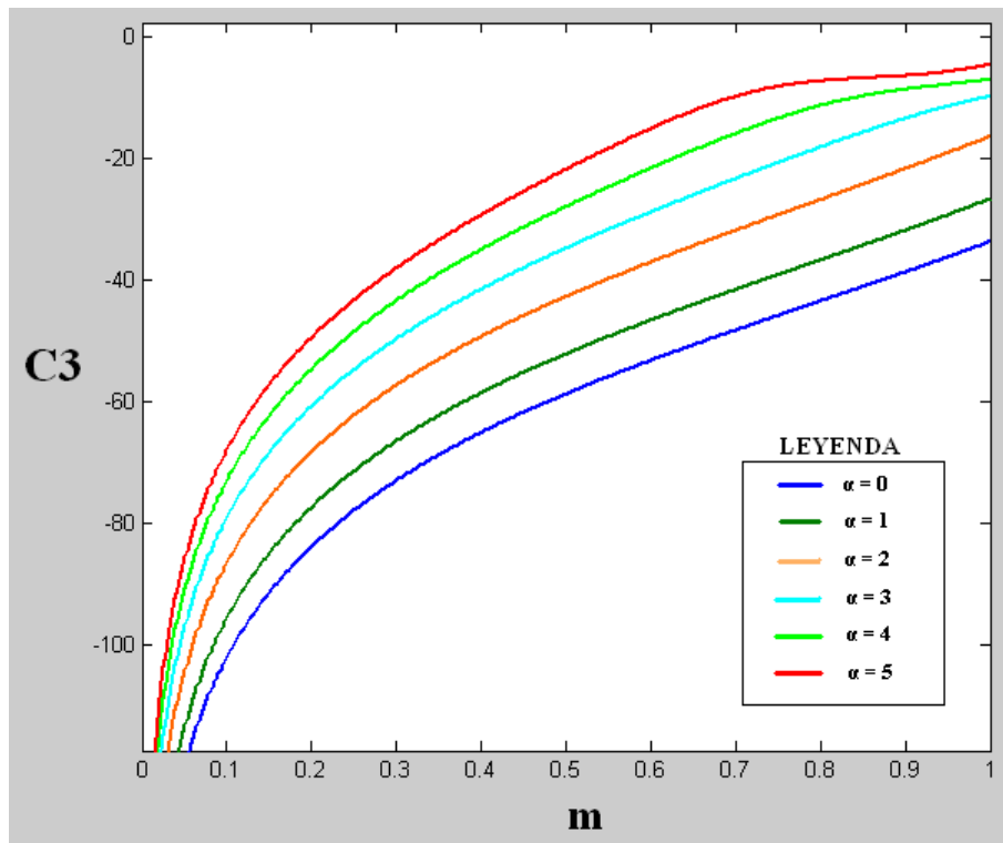
Figura 4.9. Amplitud tercer armónico vs m para valores de \alpha comprendidos entre 0 y 5,
