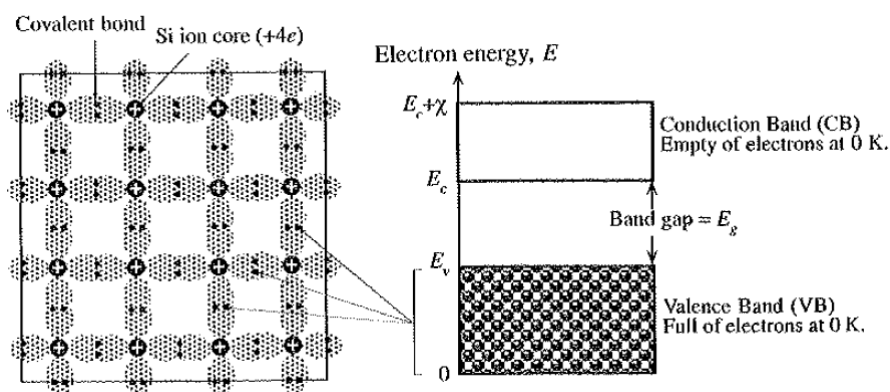
Figura 1.1. Esquema simplificado de una región de un cristal de silicio. Cuando los electrones están ligados a los átomos del material, decimos que están en la banda de valencia.
