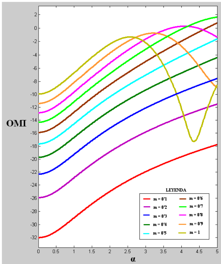
Figura 4.1. OMI vs \alpha para valores de m comprendidos entre 0 y 1, empleando 10 coeficientes de Taylor.
