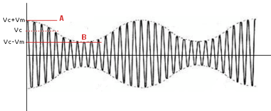
Figura 2.1. Portadora modulada, y representación de la envolvente.
