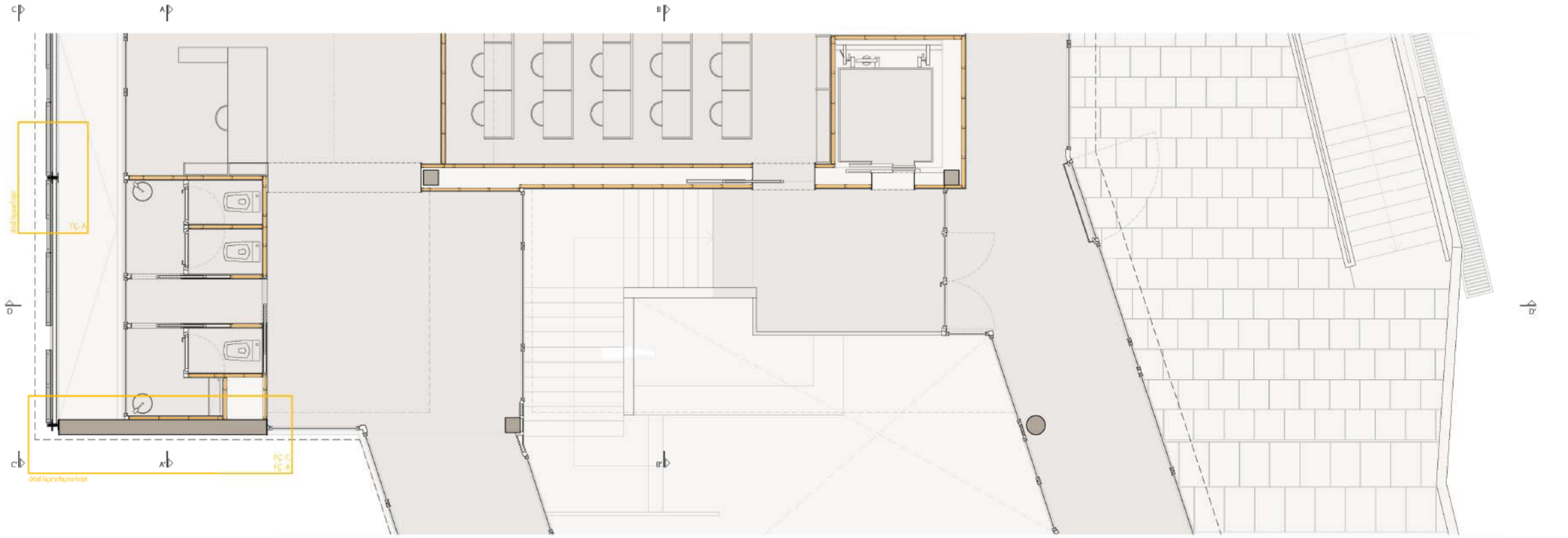
PLANTA PRIMERA E: 1/50
