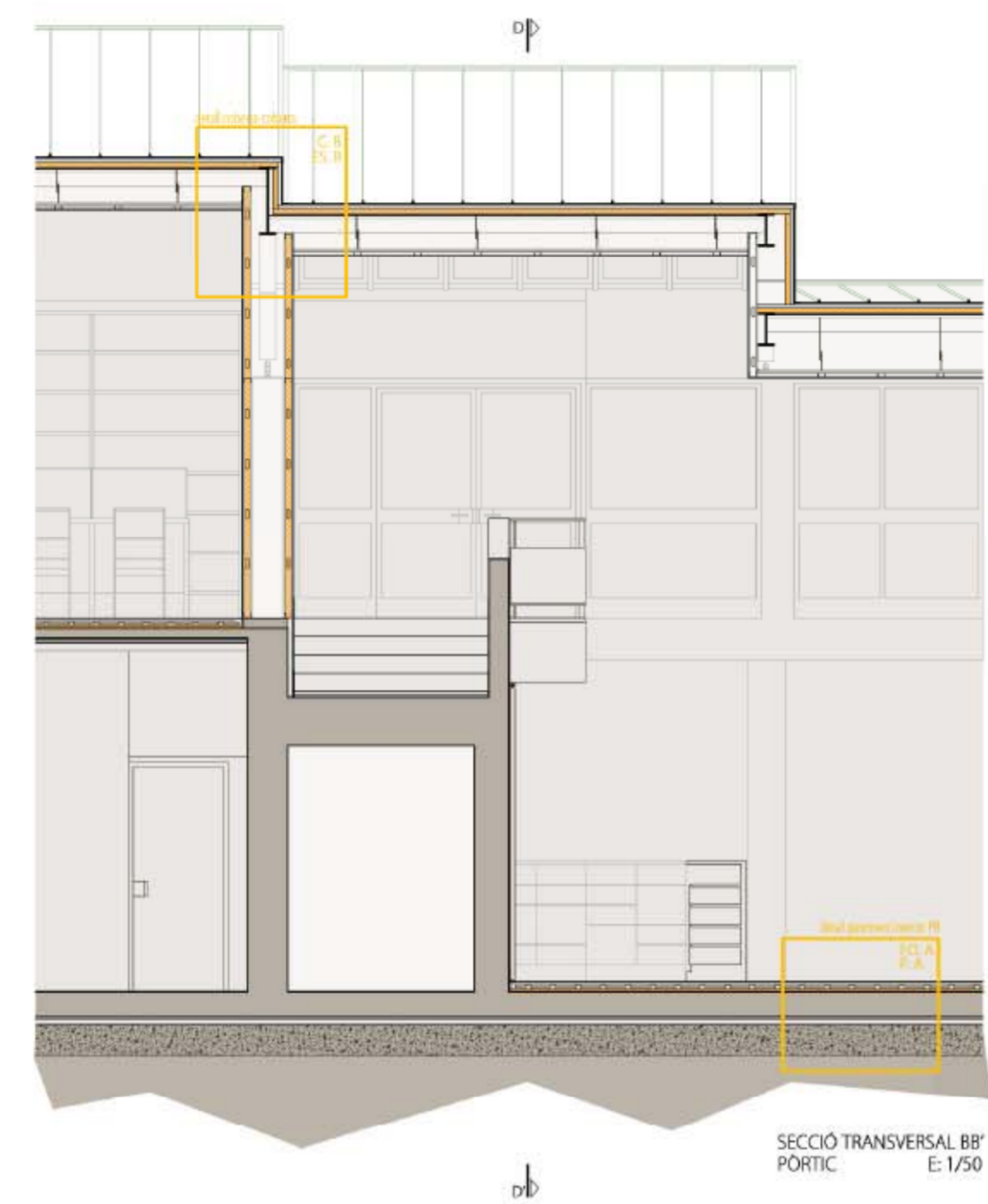
SECCIÓ TRANSVERSAL AA' PORTIC E: 1/50
