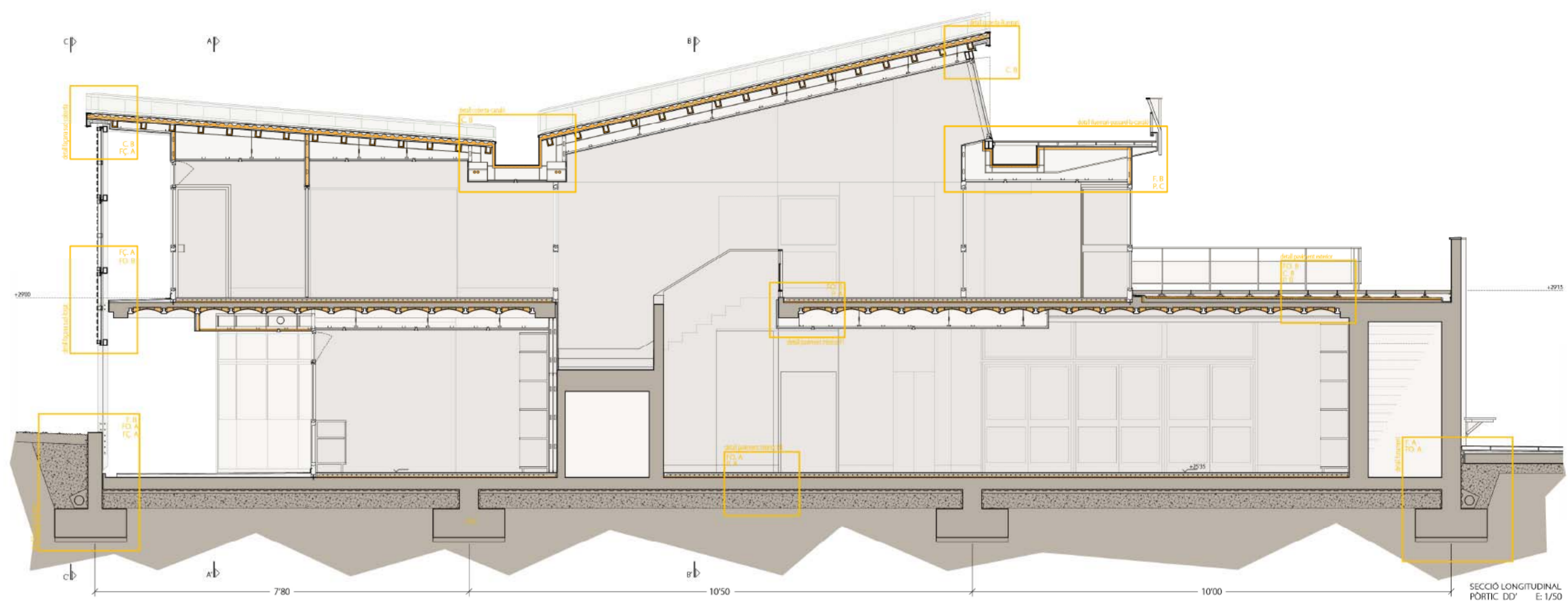
SECCIÓ TRANSVERSAL BB' PORTIC E: 1/50
