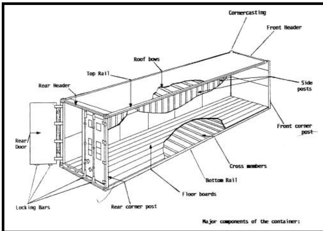
Figura 5: esquema parts del contenidor
