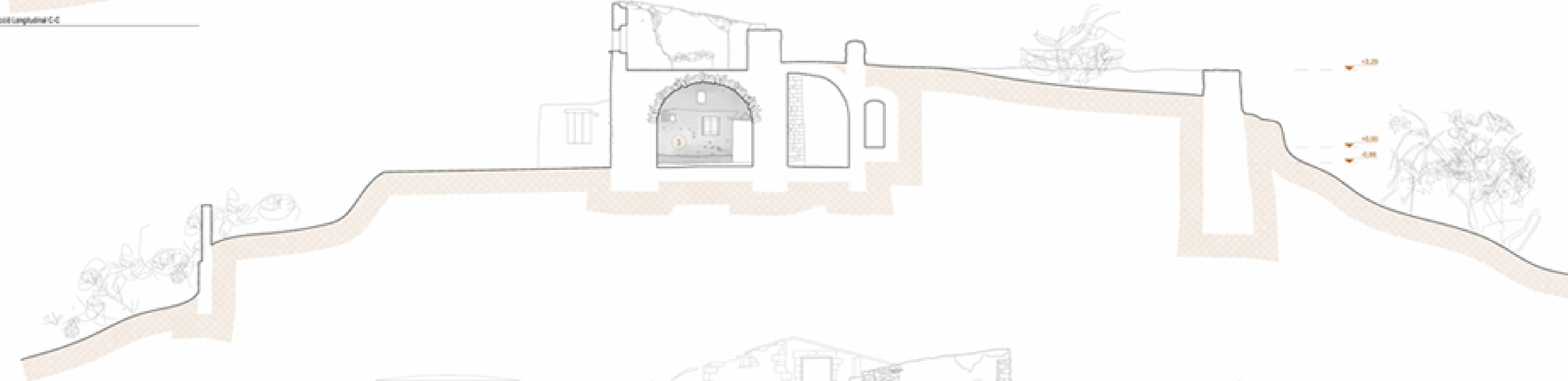
Algal·Seccó Longitudinal B-B
