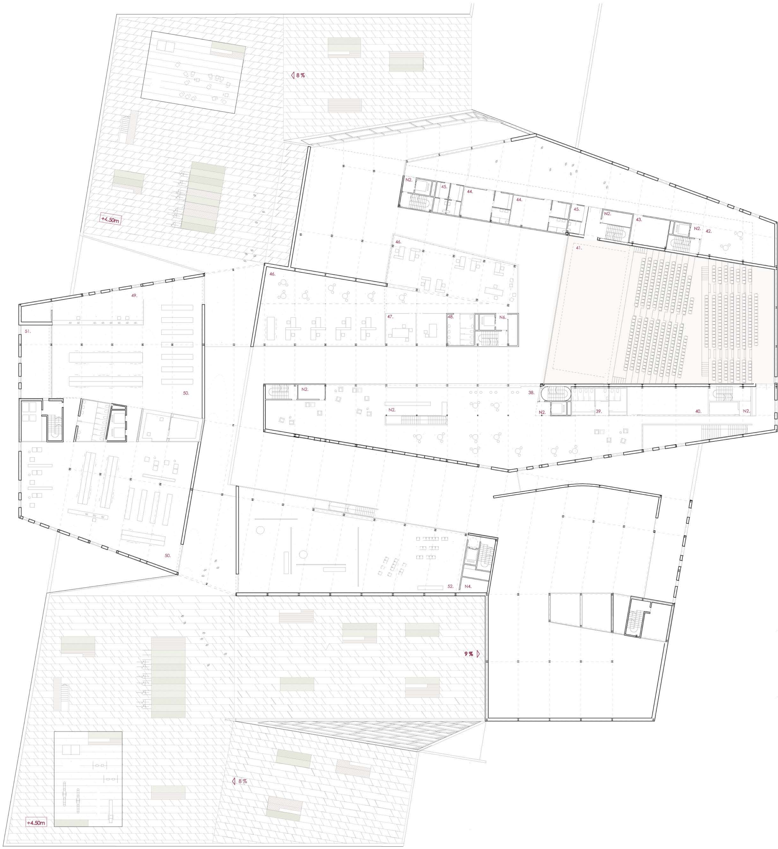
PLANTA PRIMERA, COTA 4.00m 0 4 16 1/300
