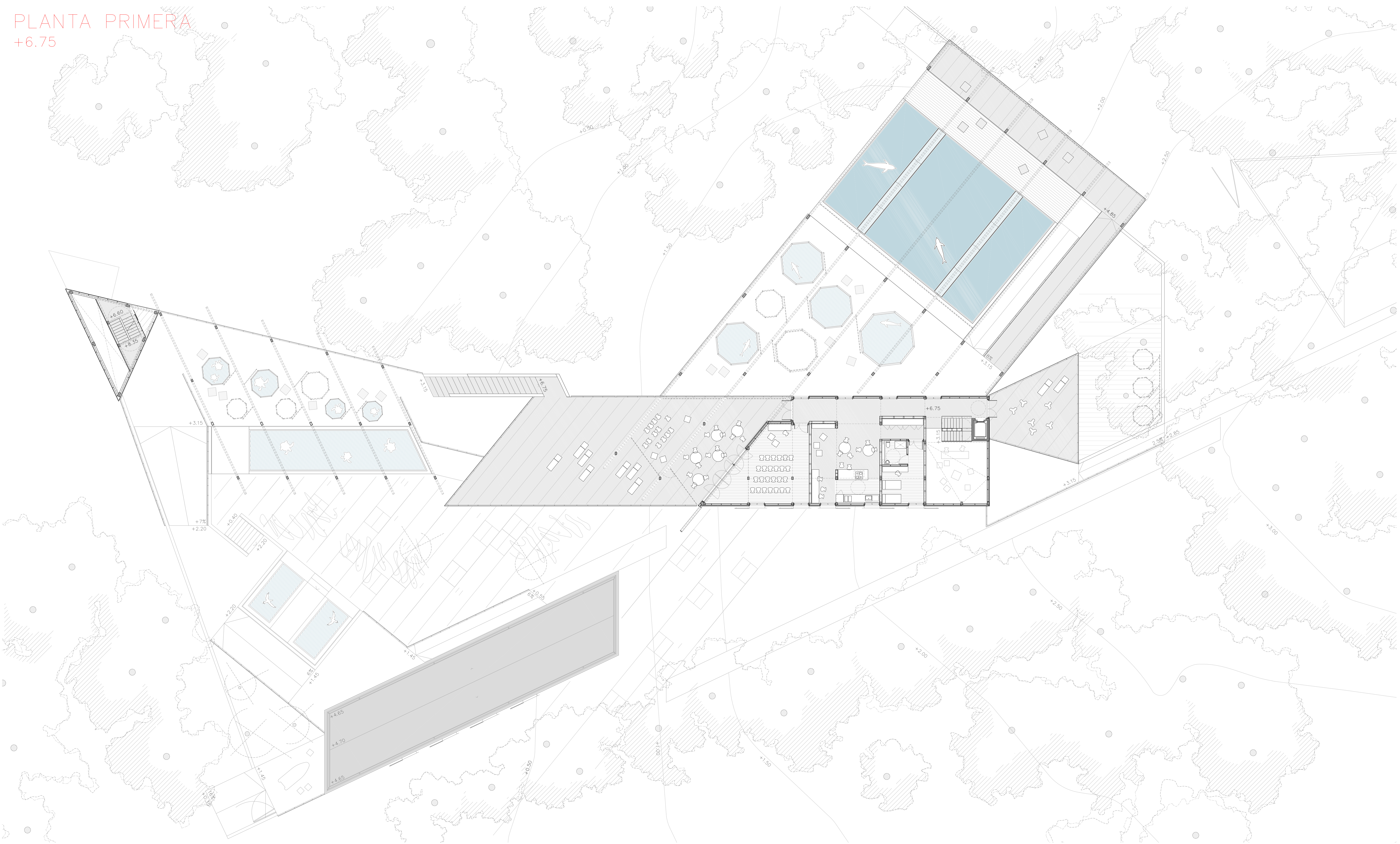
E 1/150 PLANTA PRIMERA – COTA +6.75
