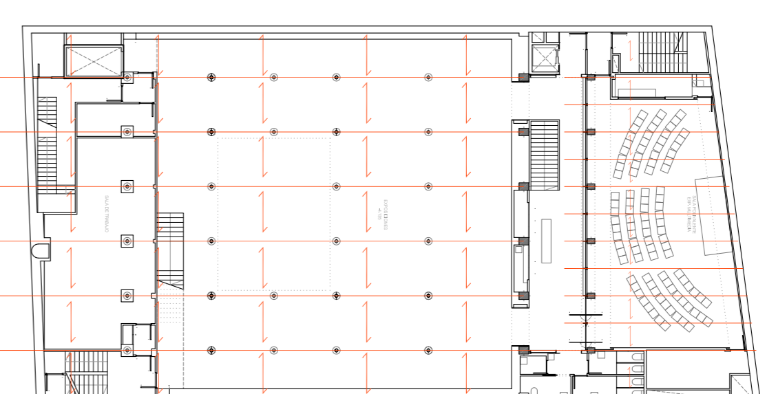
ESQÜEMA ESTRUCTURAL
