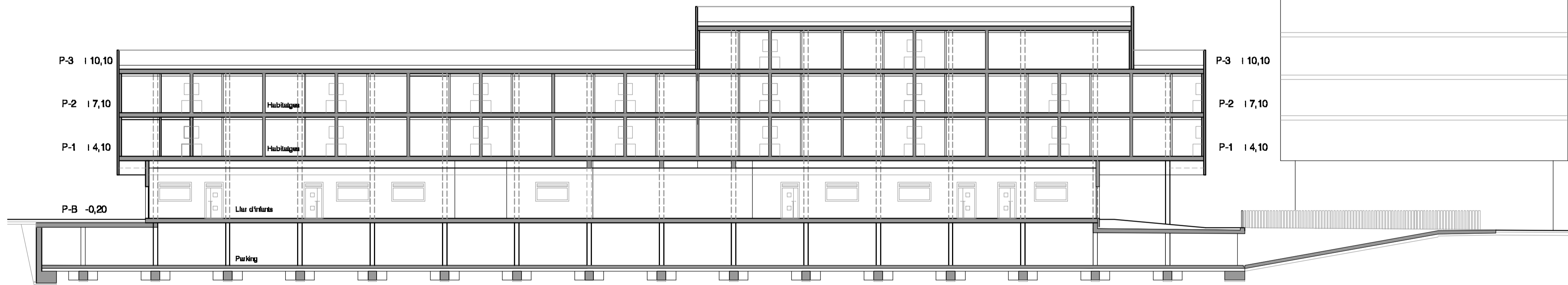
S-L1 Secció longitudinal
