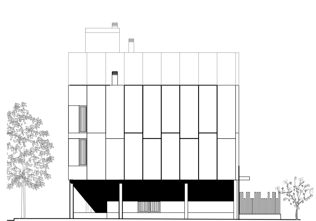
Alçat Sud-oest
