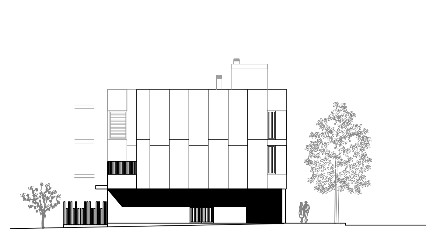
Alçat Nord-est c/Casanova
