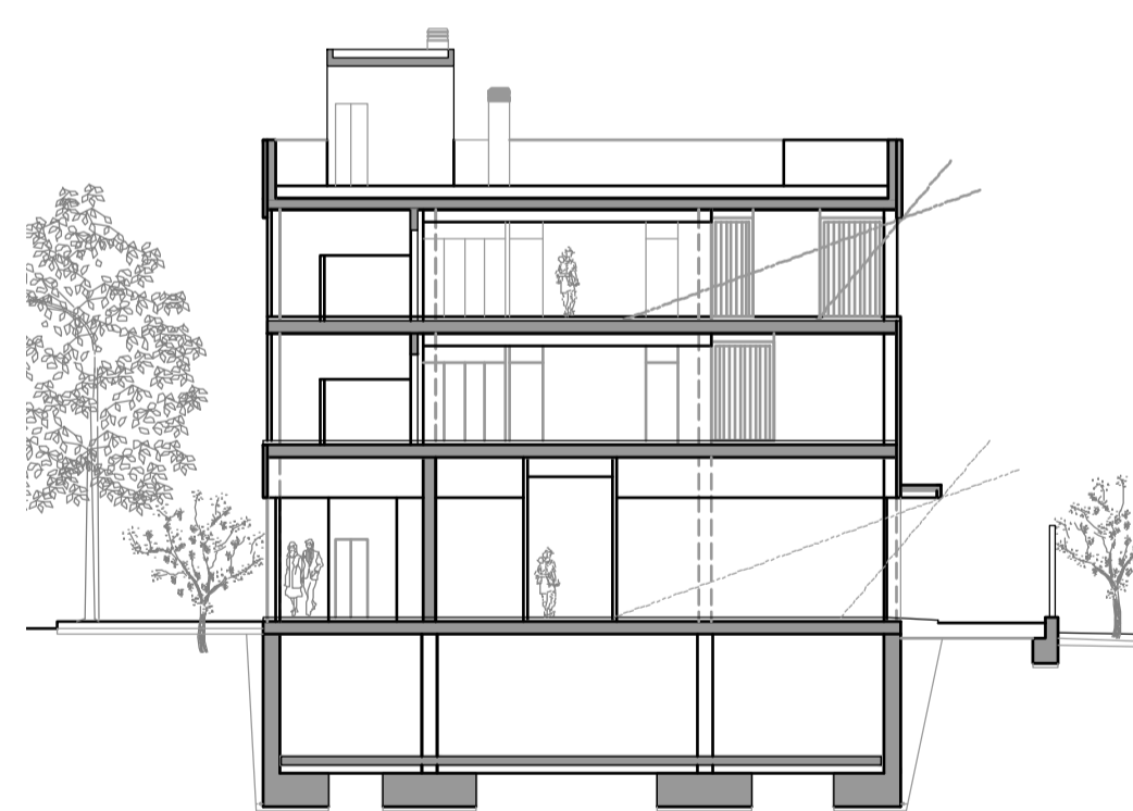
S-T1 Secció transversal
