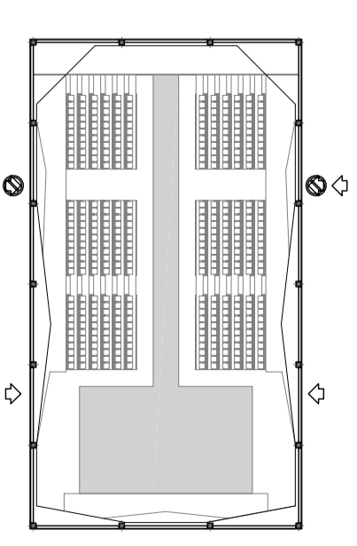
Pasarela 396 espectadors 146,90 m 2 escènics
