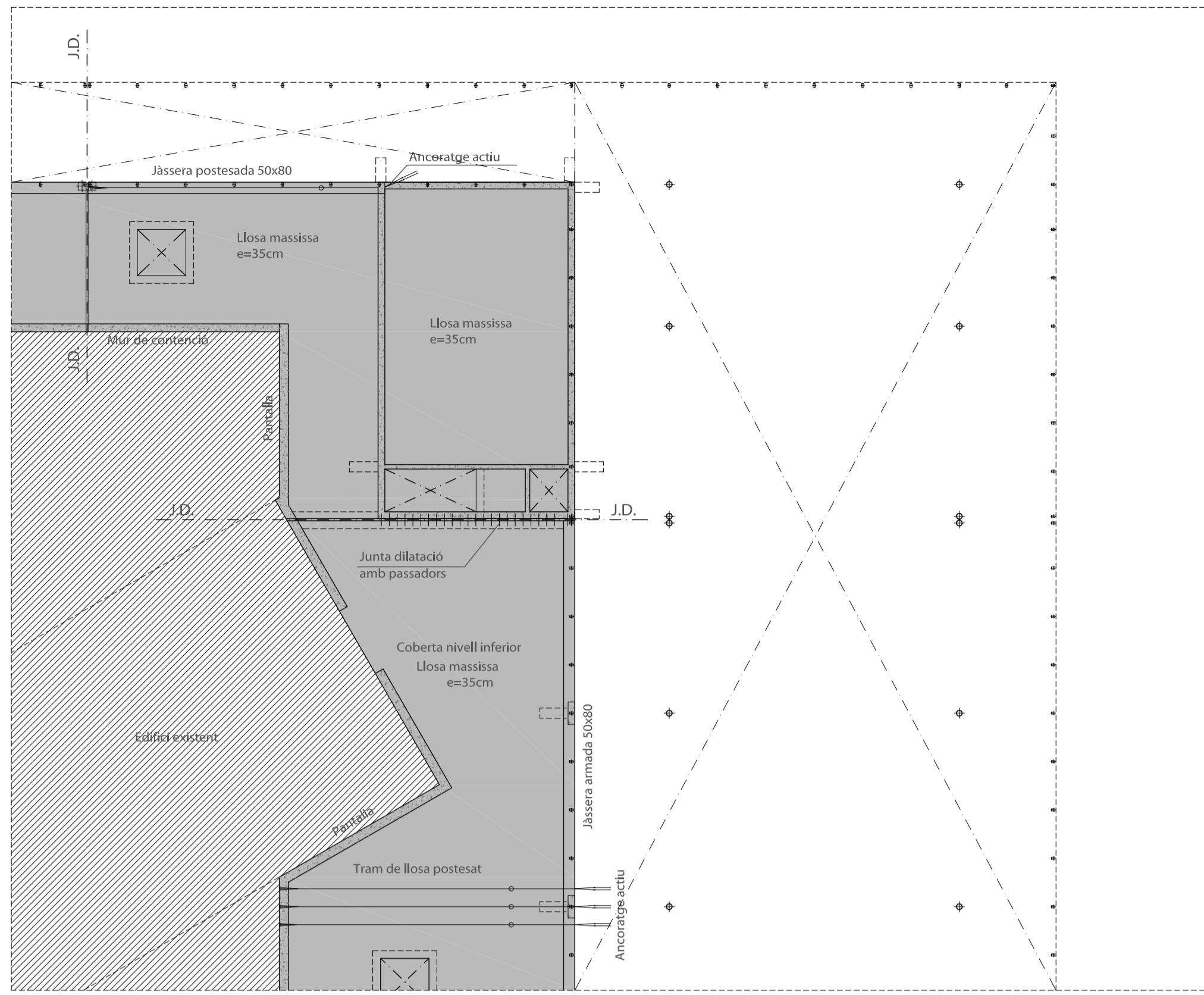
COBERTA NIVELL INFERIOR E:1/200
