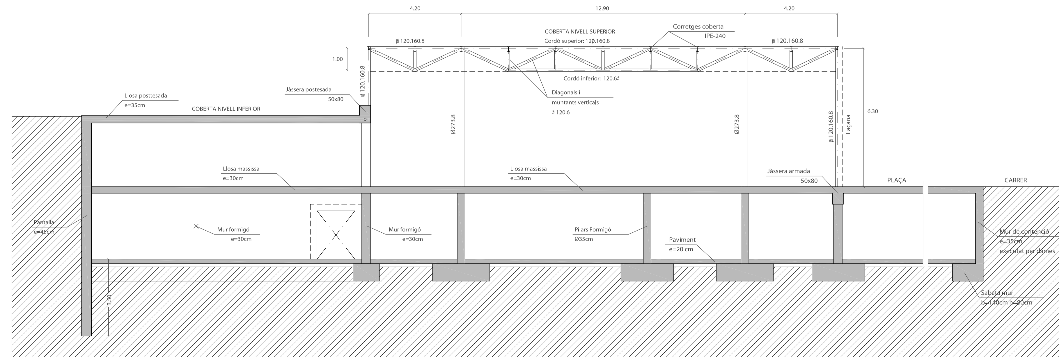
SECCIÓ TIPUS 1 E: 1/100
