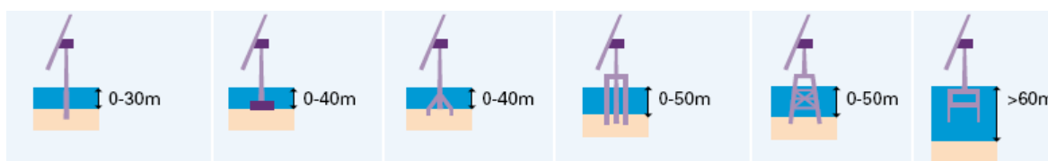
Fig. 5.2. S'adjunta l'interval de profunditat per a cada fundació. Per ordre d'esquerra a dreta: monopiló, fundació per gravetat, tripode, tripiló, jacket i flotant. [Font: BWEA]
