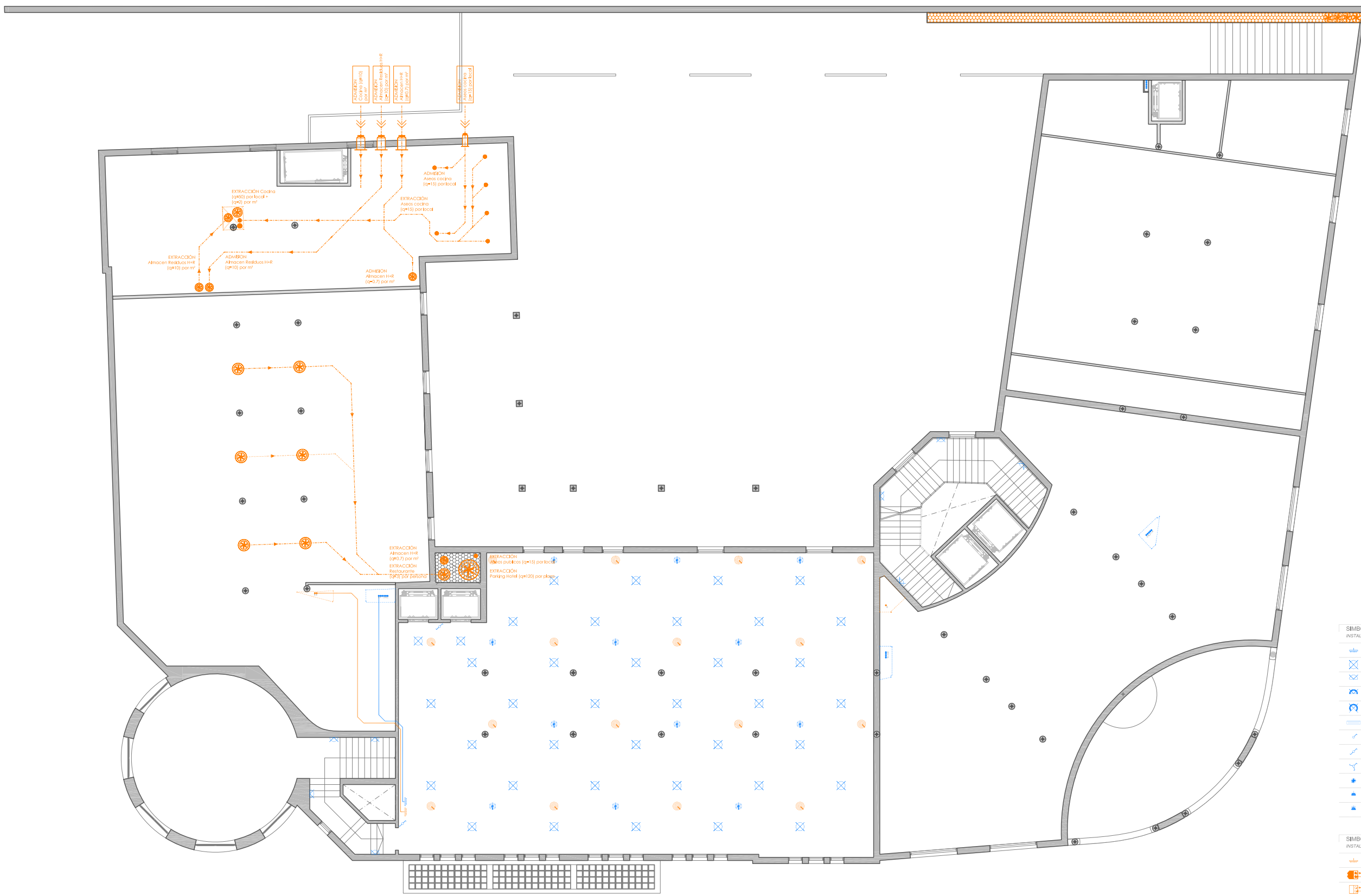
PLANTA ENTRESUELO ESCALA 1:200
