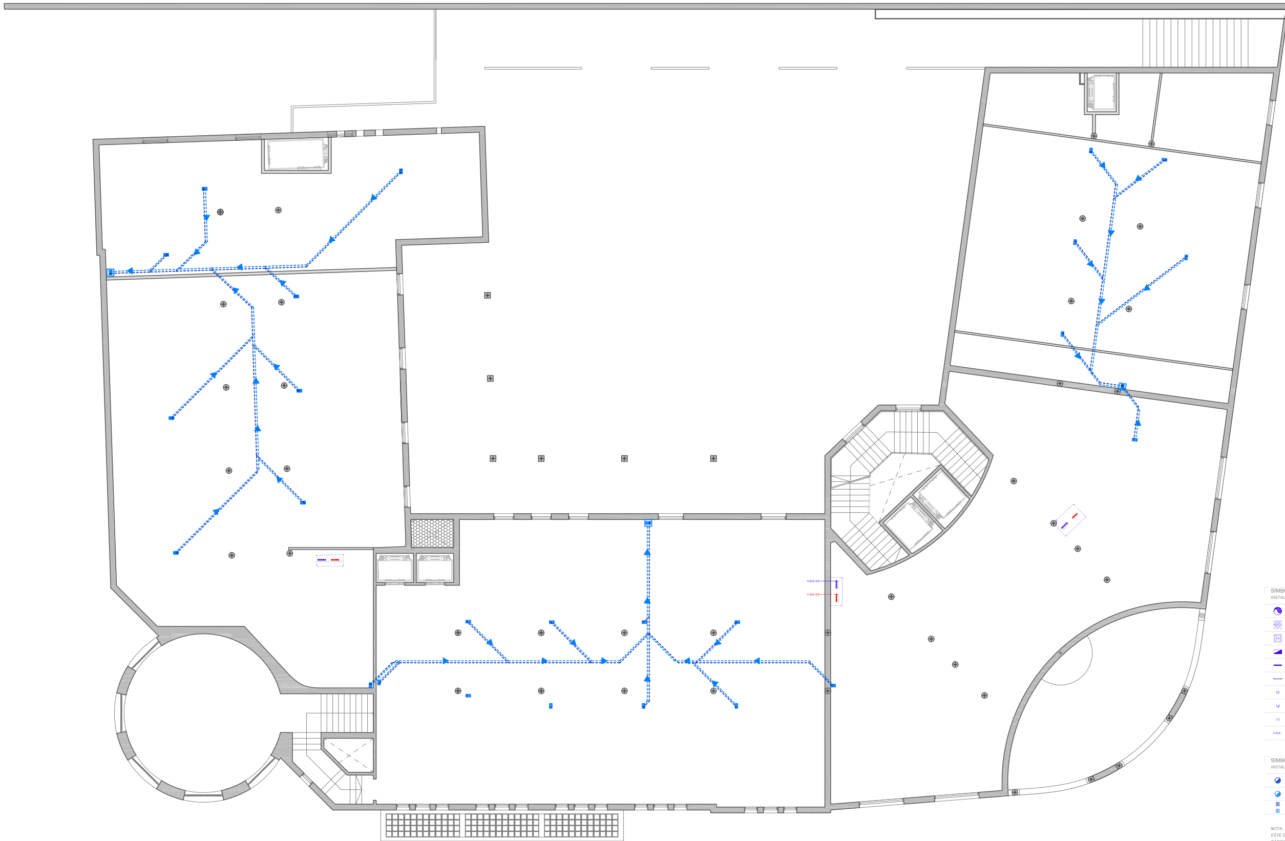
PLANTA ENTRESUELO ESCALA 1:200
