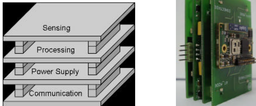
Figura 2: Nodo red de sensores CEI
