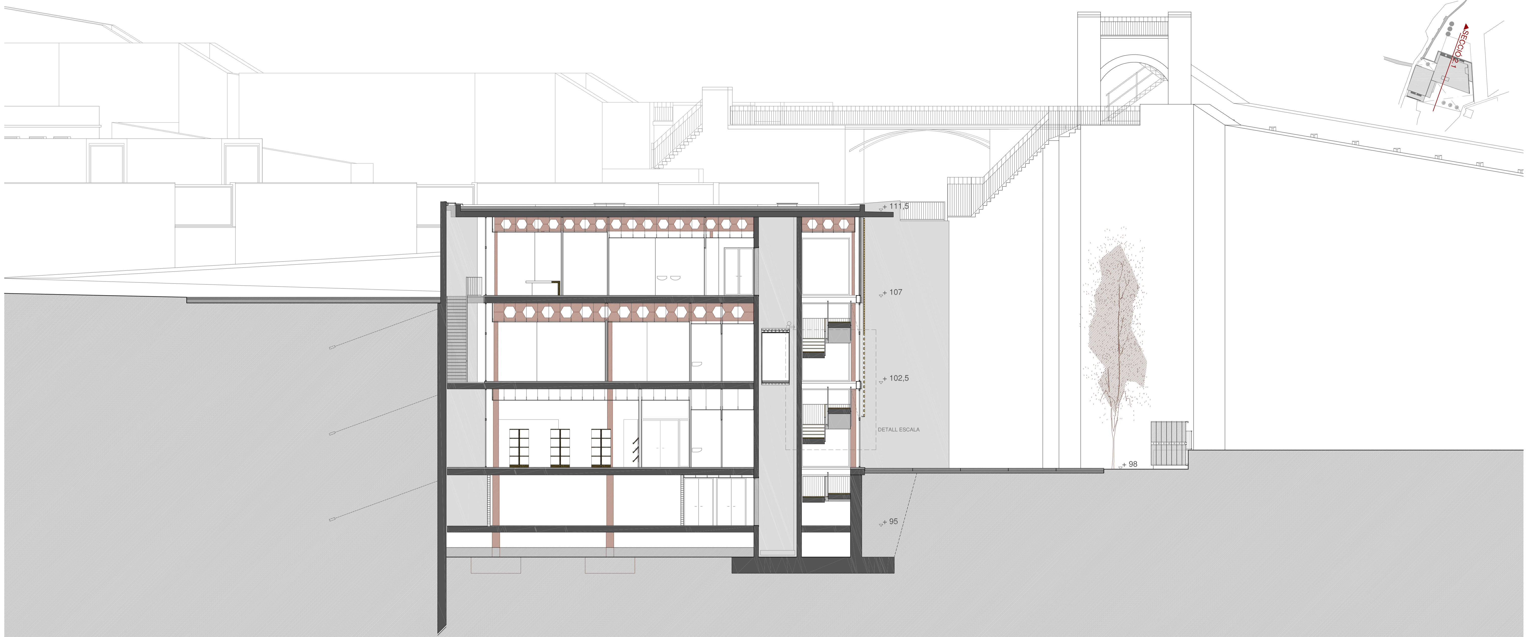
SECCIÓ 2.1
