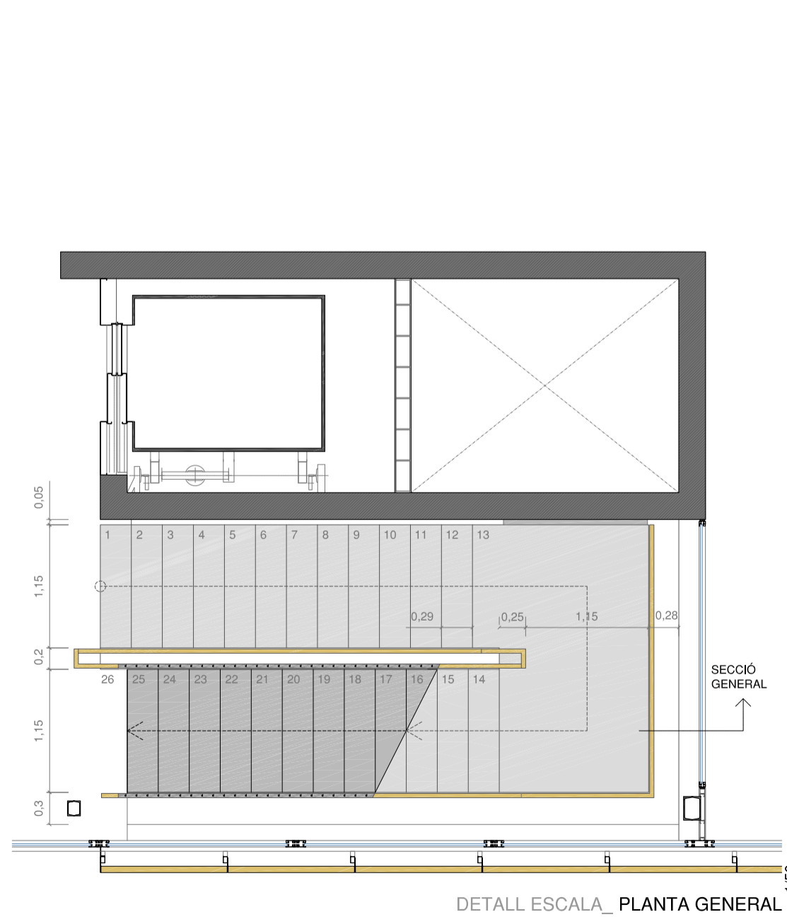
DETALL ESCALA_PLANTA GENERAL 1/50
