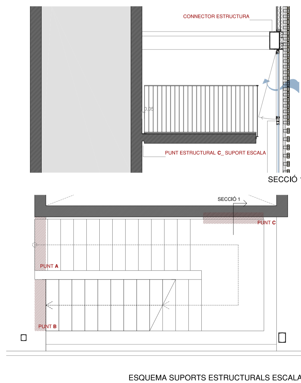
ESQUEMA SUPORTS ESTRUCTURALS ESCALA 1/50
