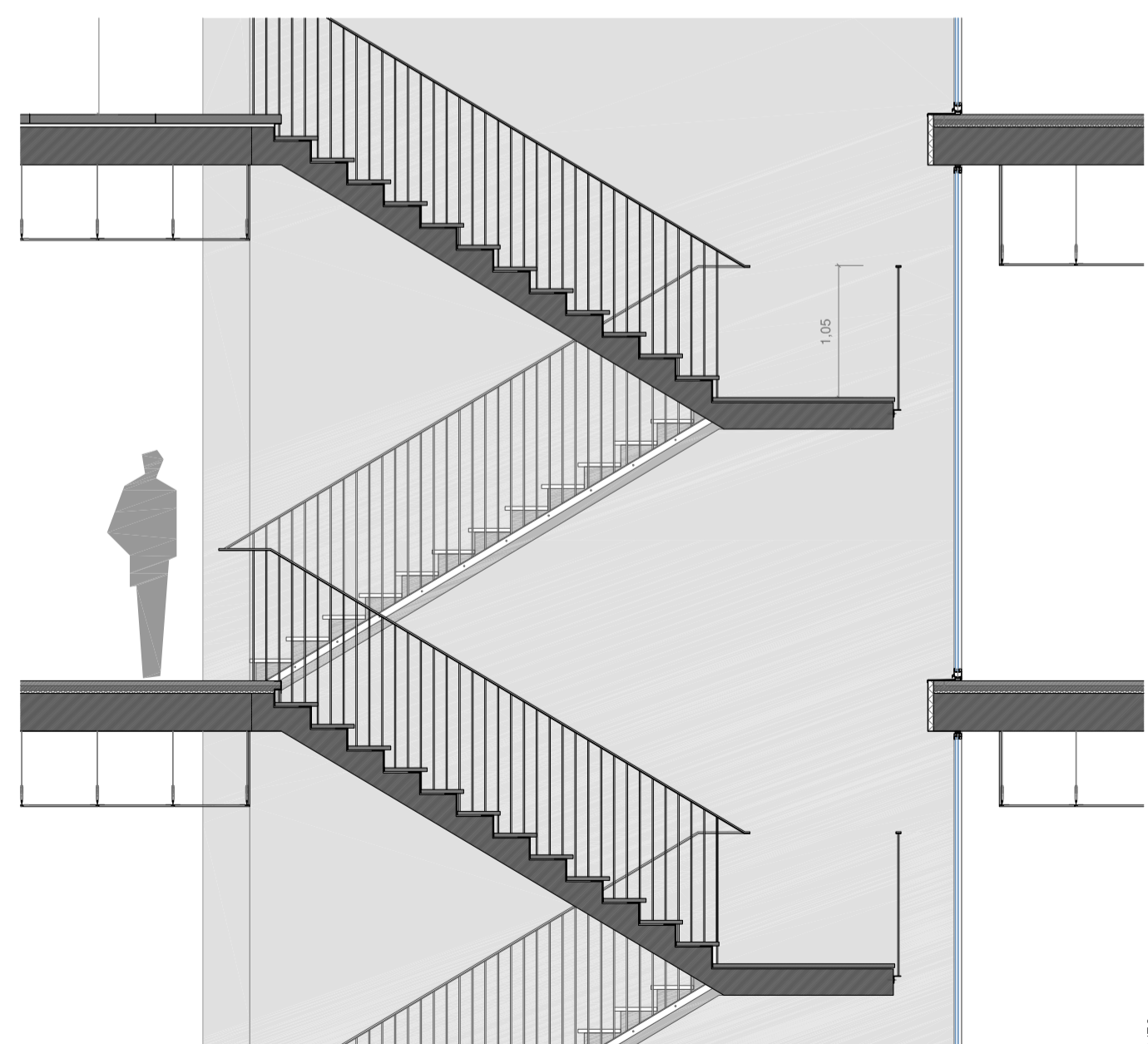
SECCIÓ GENERAL 1/50
