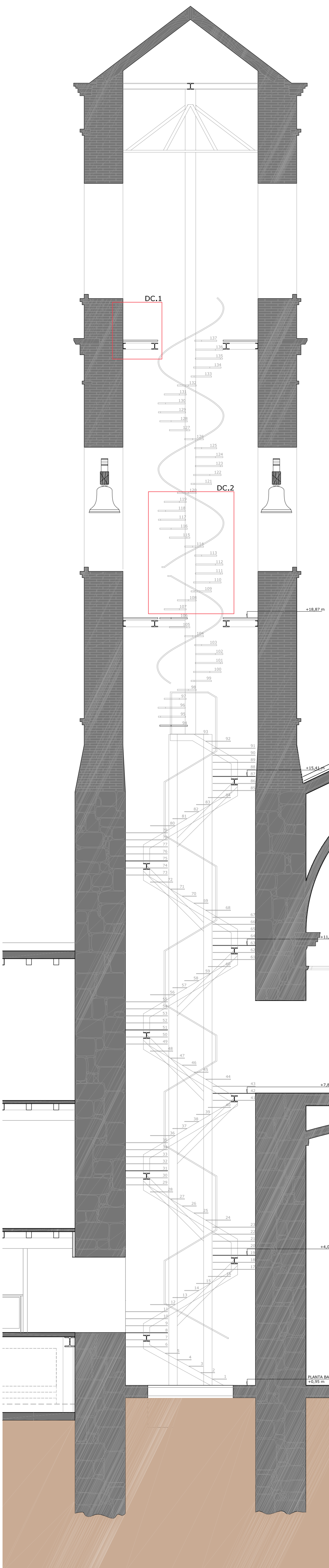
SECCIÓ 1 E (1/50) L'ESTRUCTURA DE L'ESCALA
