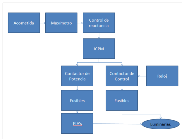
Esquema 3.3. Bloques funcionales general
