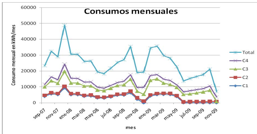
Gráfica 3.1. Consumos correspondientes a las zonas diferentes zonas
