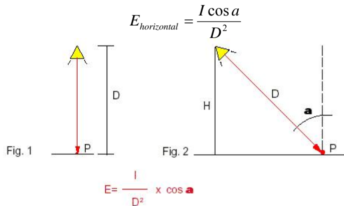
Fig. 2.4. Ley del coseno de incidencia
