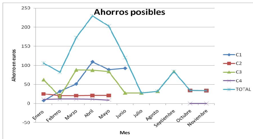
Gráfica 3.3. Posibles ahorros aplicando correctamente la Tarifa contrada
