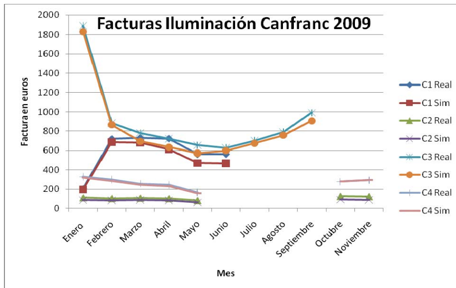
Gráfica 3.2. Facturación en 2009 comunicada por la compañía en los diferentes circuitos.
