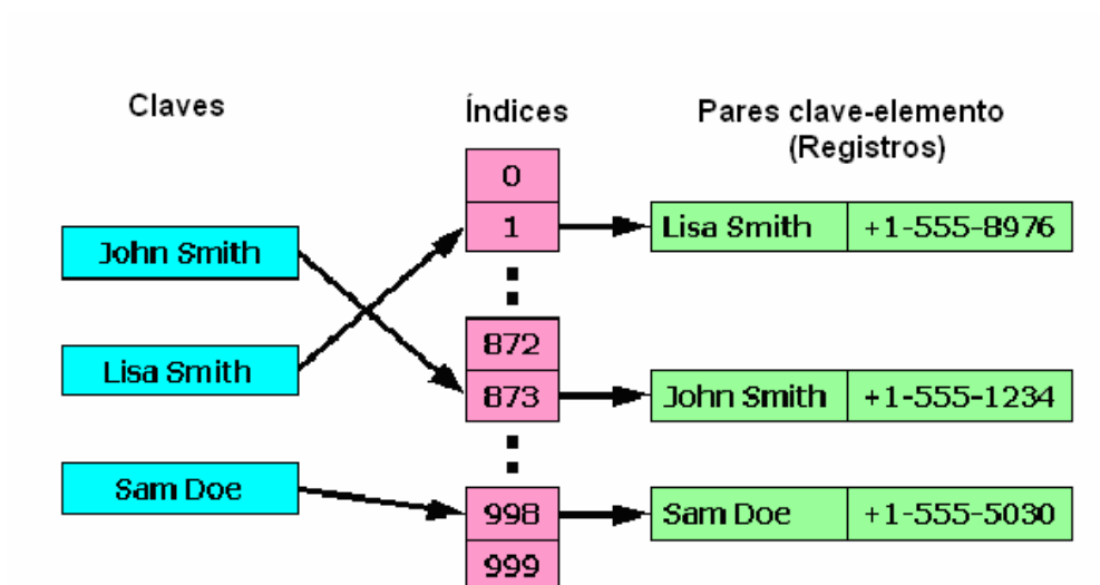
Fig 2.6 Esquema de una tabla de Hash
