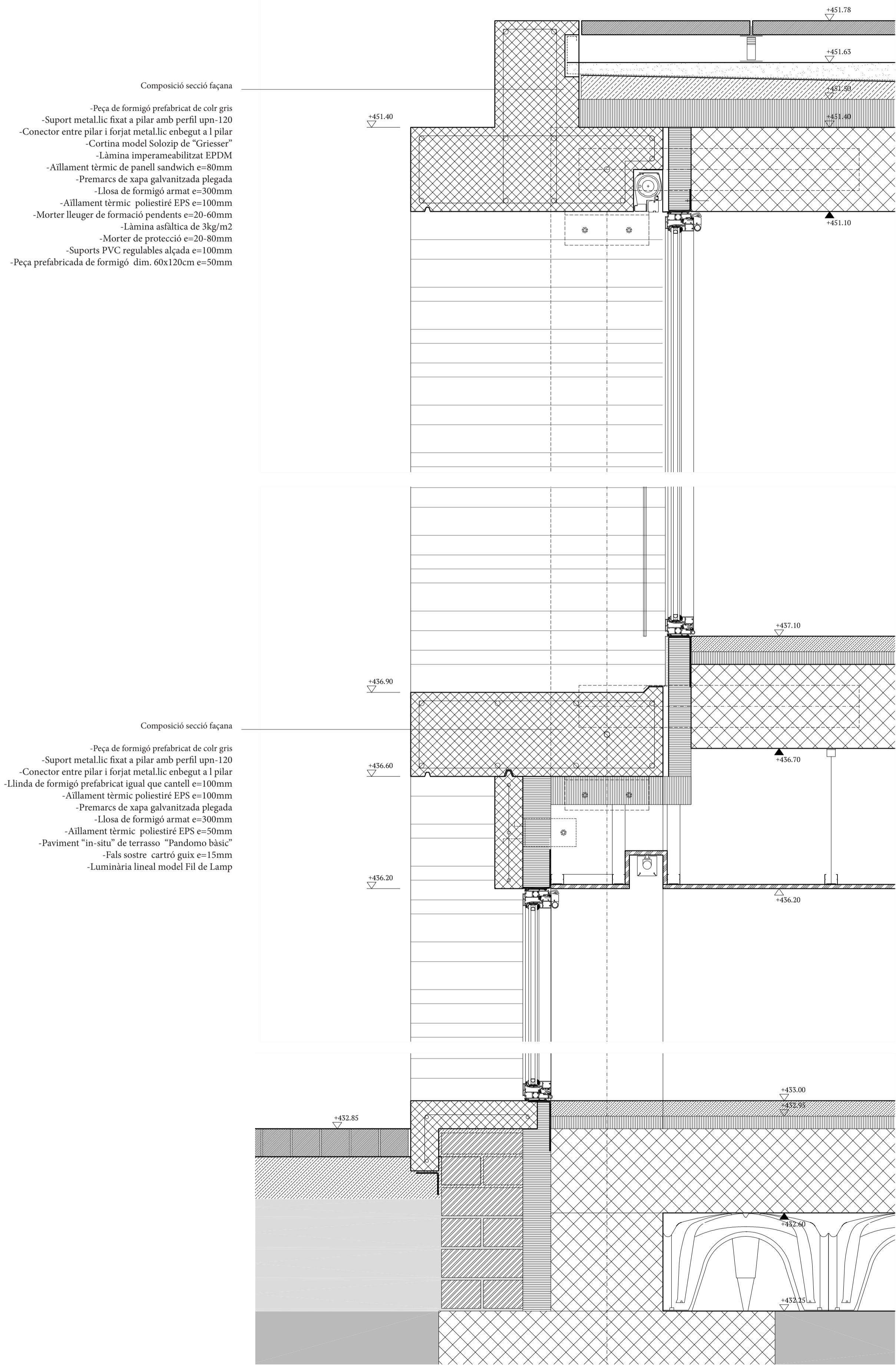
Secció vertical tipus amb finestra al sòcol escala: 1/10
