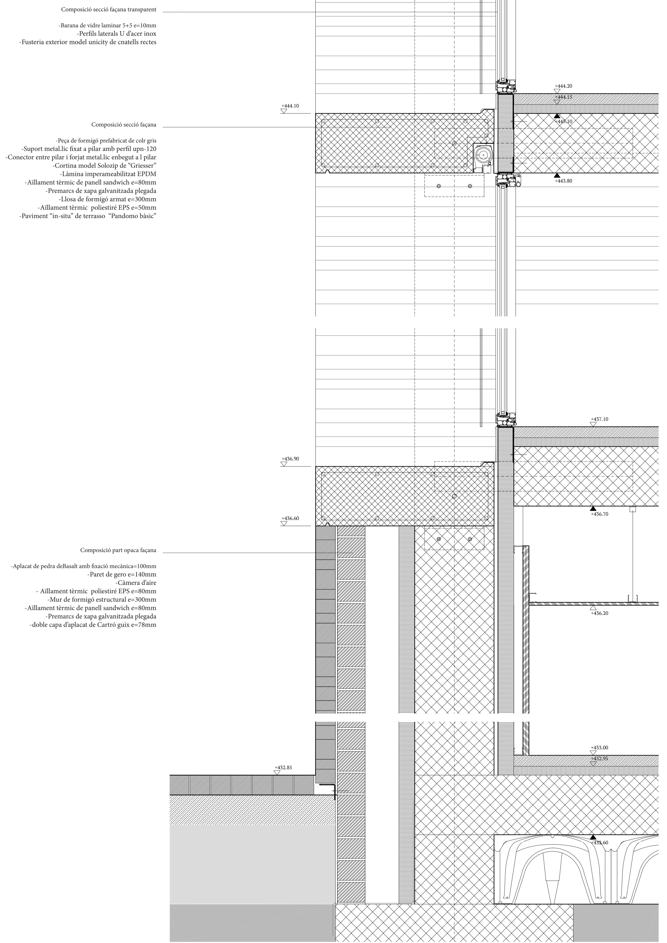
Secció vertical tipus escala: 1/10
