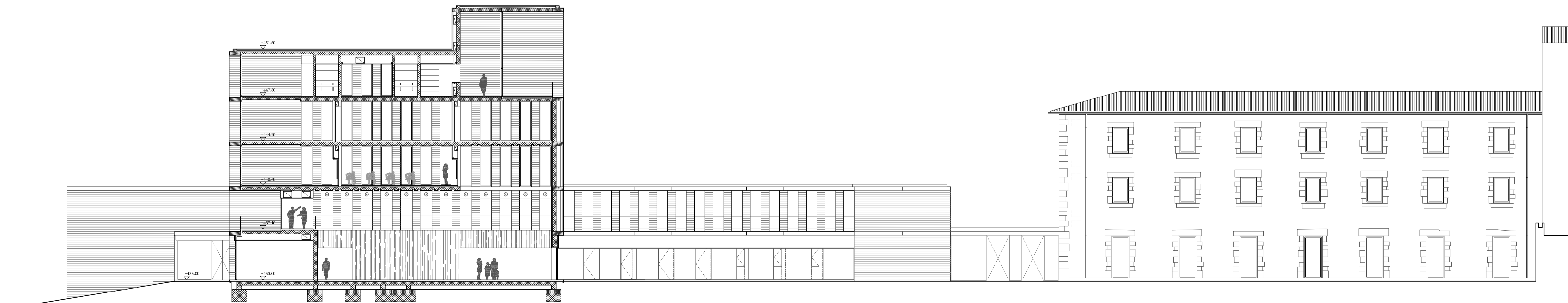
Secció longitudinal vestibul escala: 1/200
