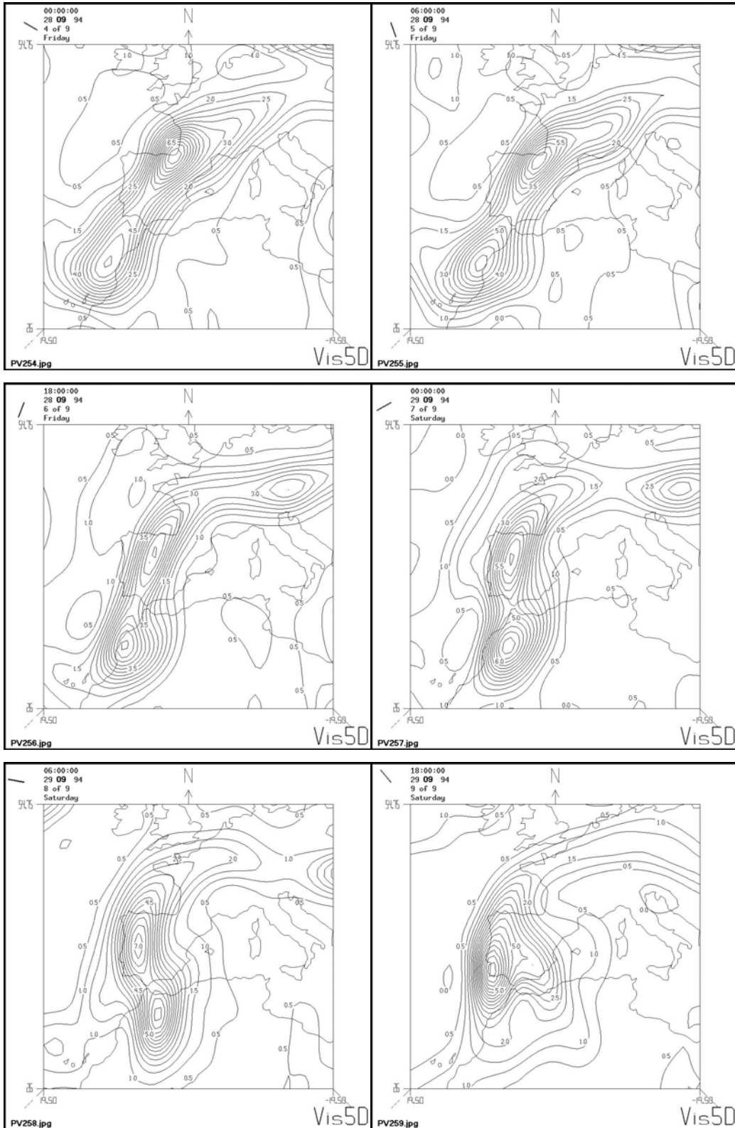
Figura 6.67.- Vorticidades potenciales en la superficie de 250hPa del episodio 28-29.09.94.
