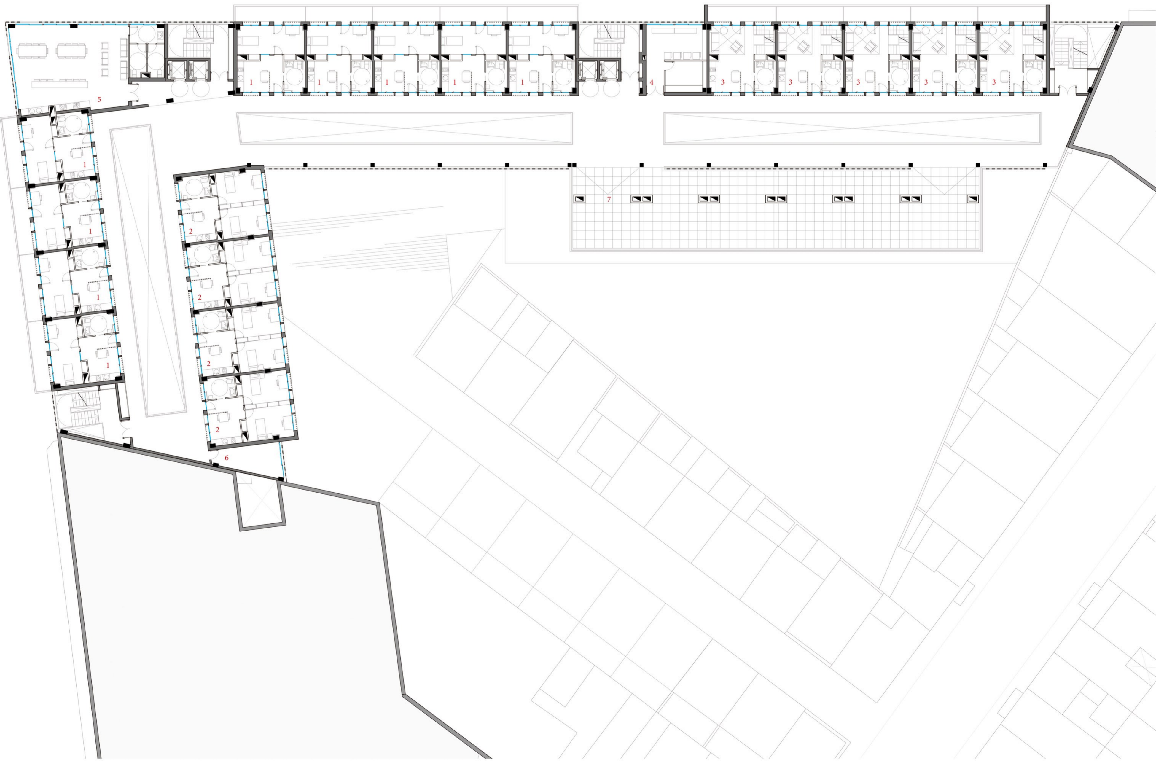
PLANTA CUARTA COTA +41'8 E 1:200
