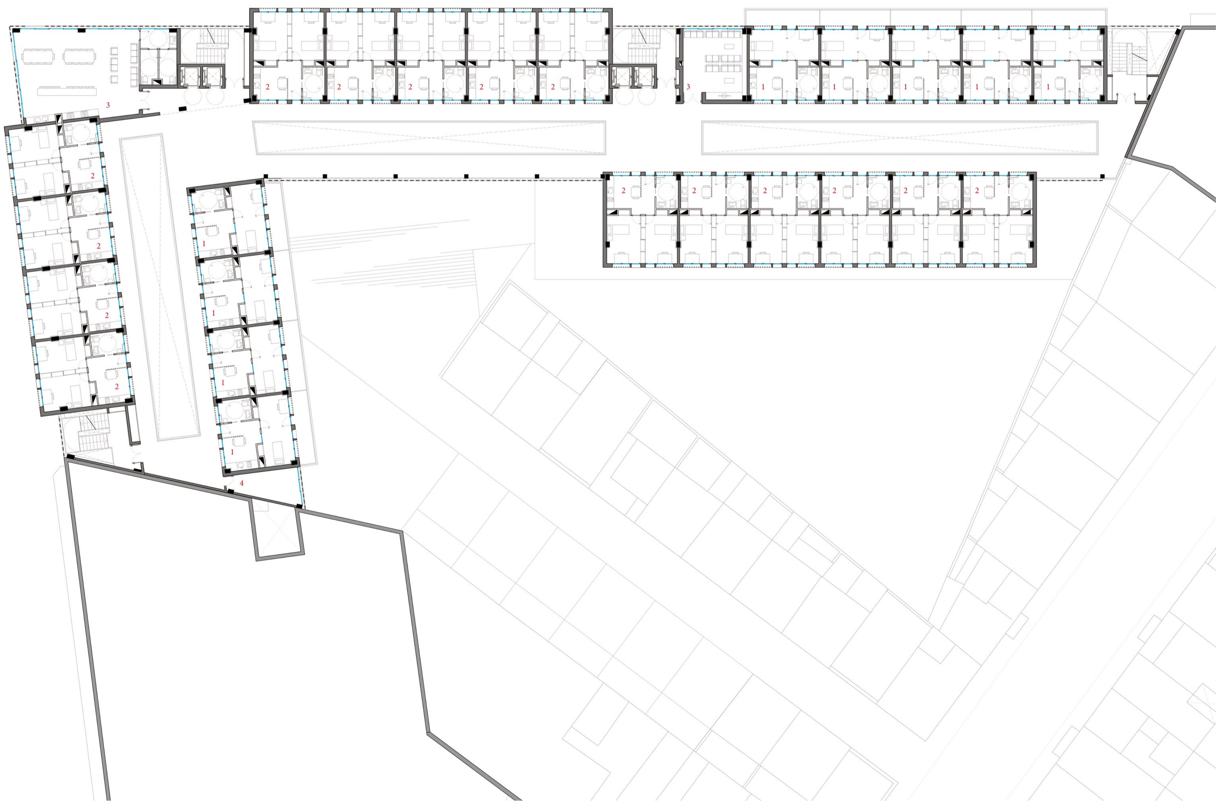
PLANTA TERCERA COTA +38'80 E 1:200
