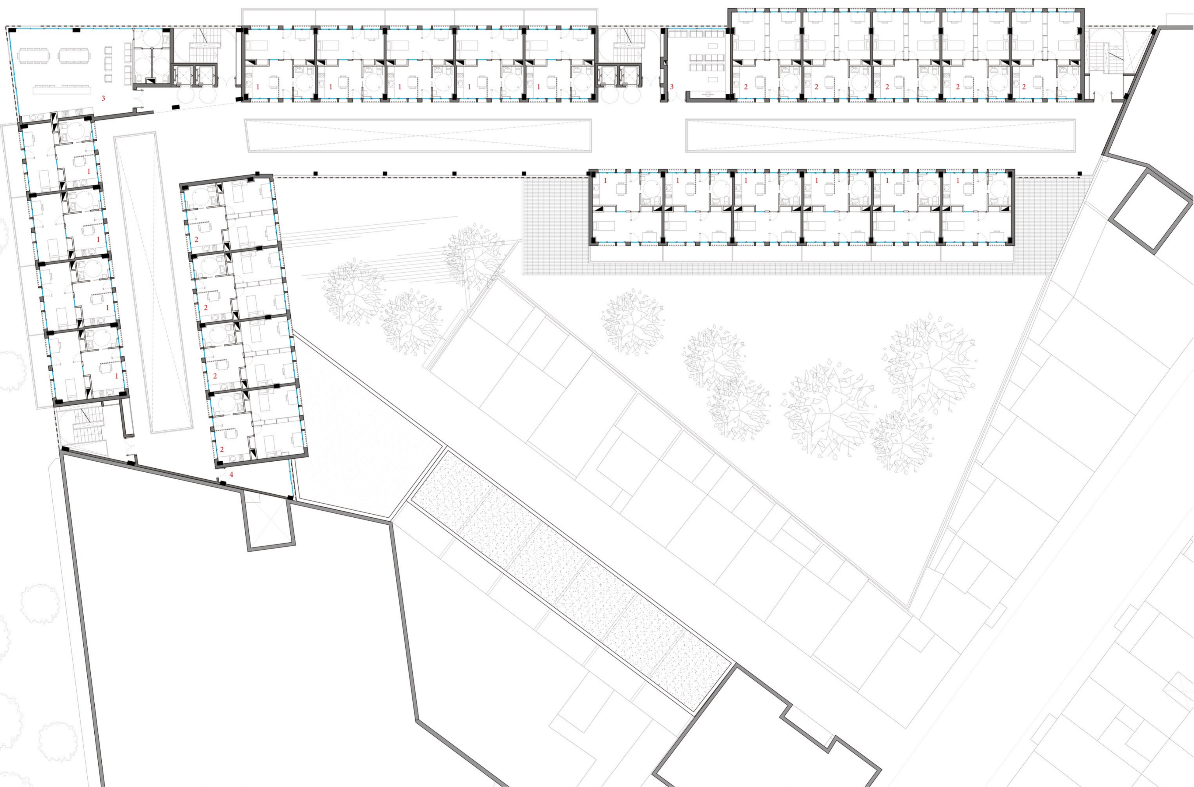
PLANTA SEGUNDA COTA +35'80 E 1:200
