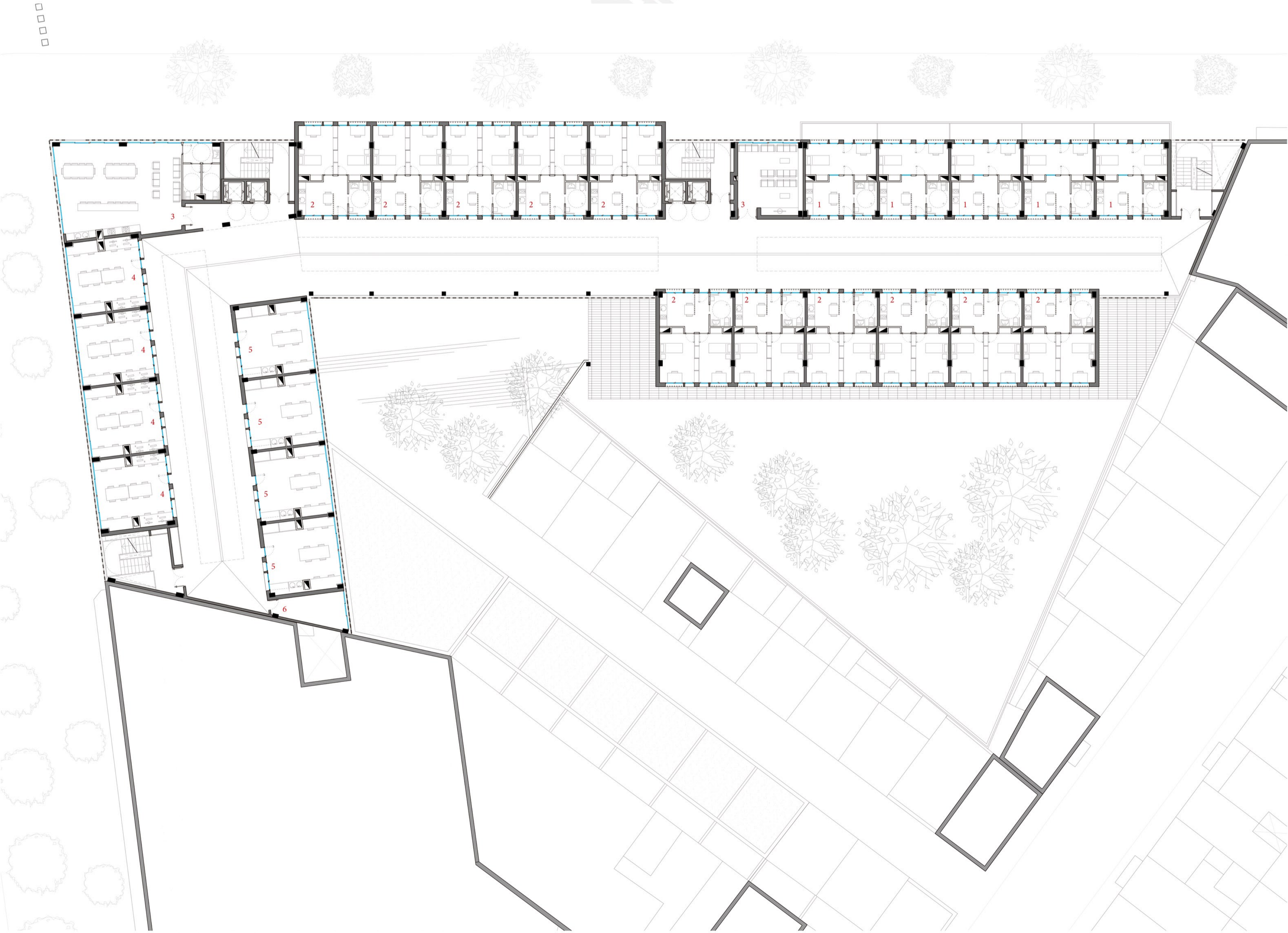
PLANTA PRIMERA COTA +32'80 E 1:200
