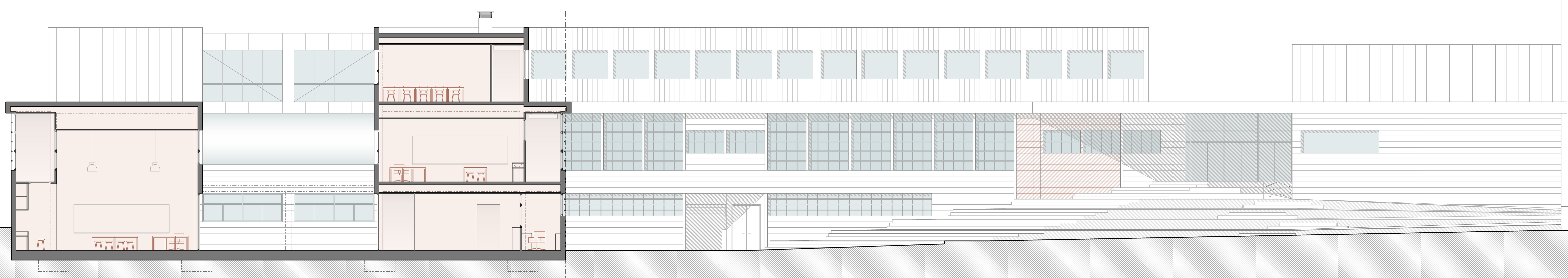
SECCIÓN AUDITORIO - NAU IVANOW
