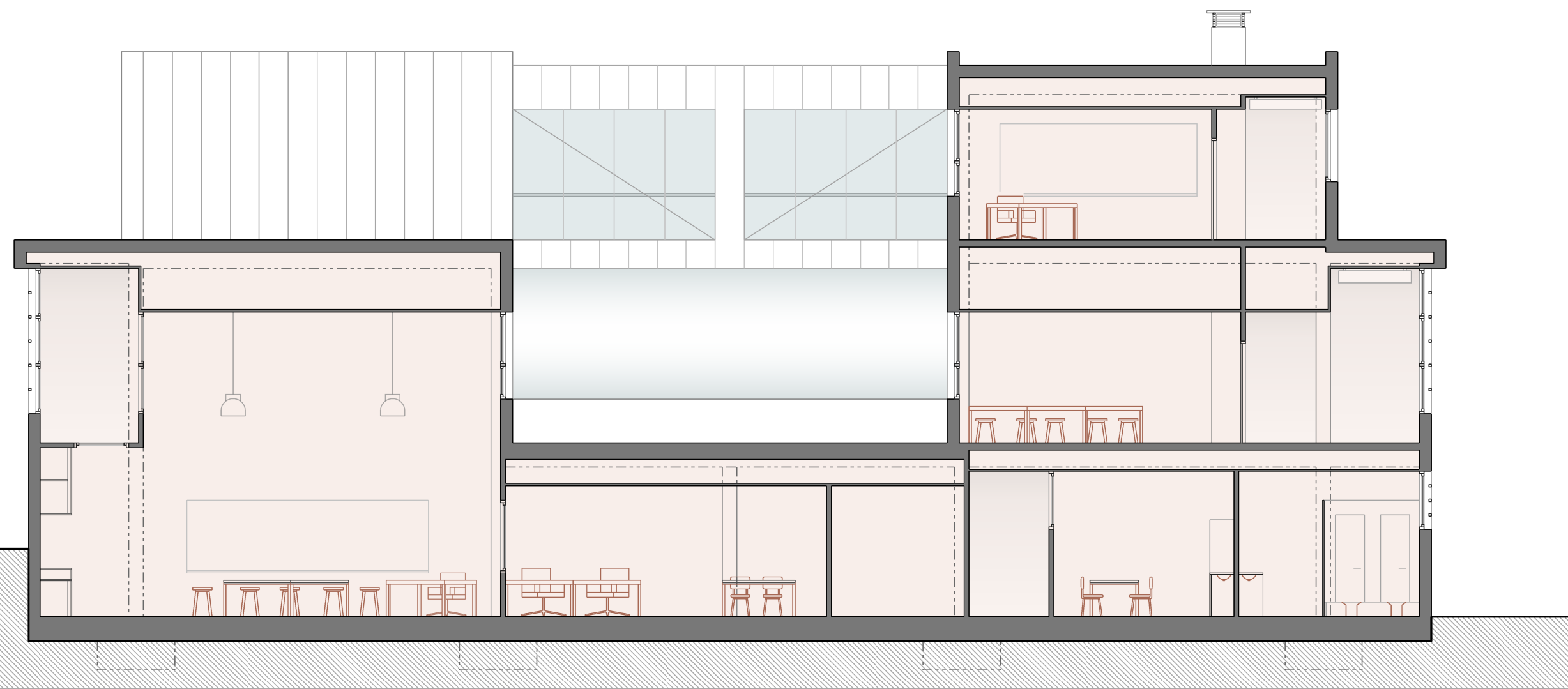
SECCIÓN TRANSVERSAL - ALZADO ACCESO PLAZA
