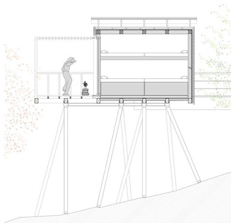
SECCIÓ TRANSVERSAL A - A'
