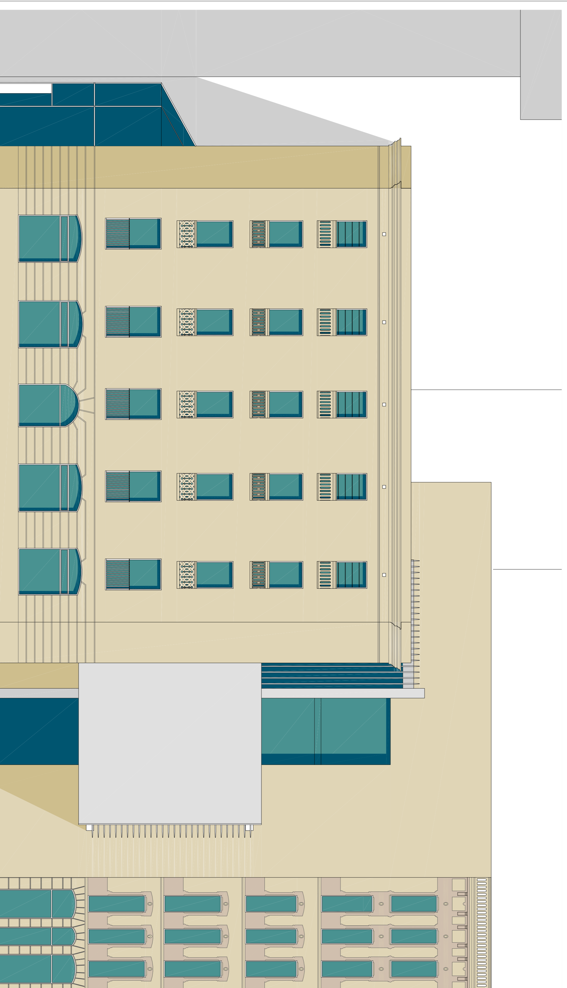
Alçat a.1 Façana a carrer Comte Urgell (sud-oest)
