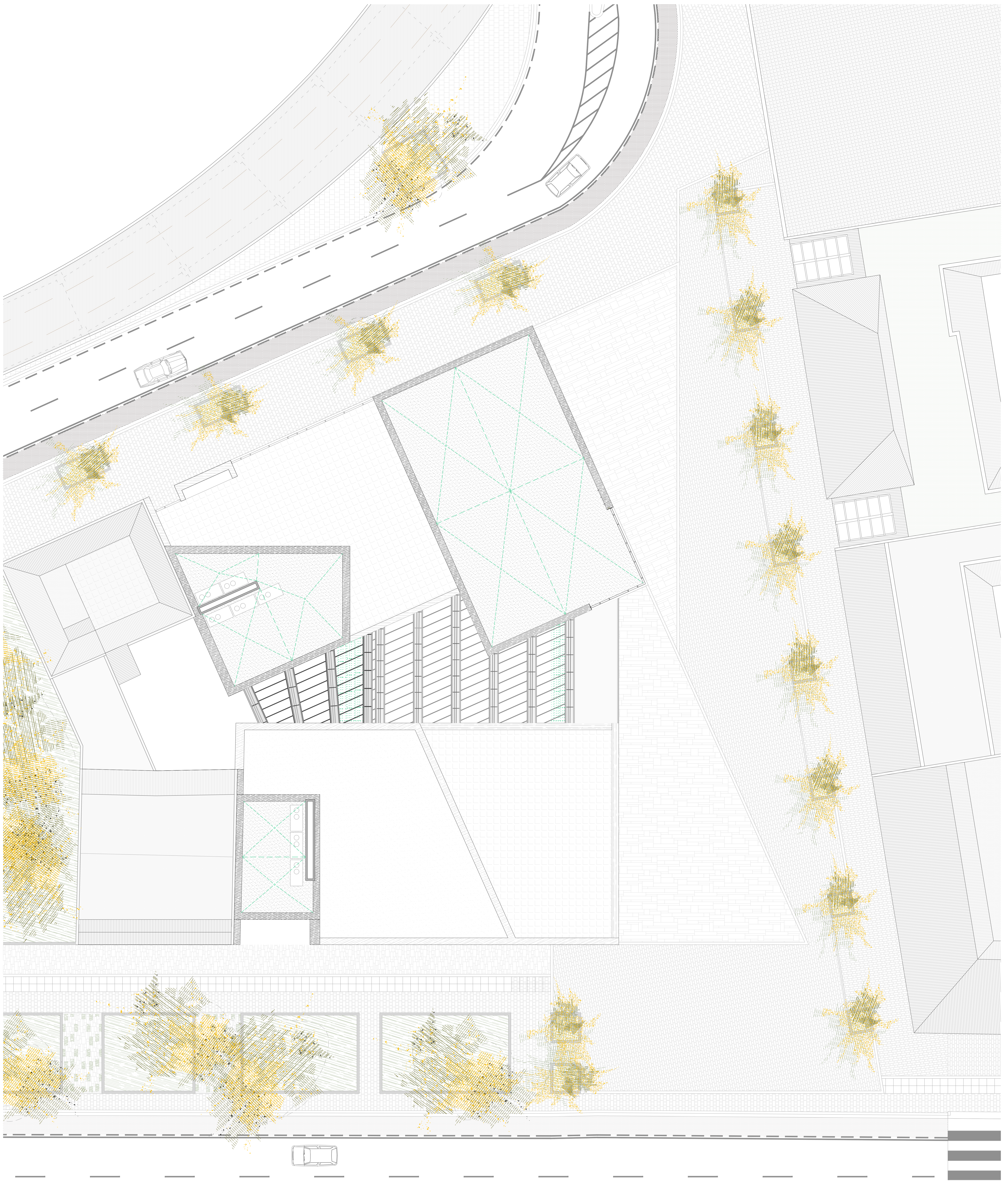
PLANTA CLERETA E-1/100
