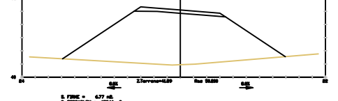
Pk=2+300 S. FINEC = 477 m. S. TORNAPLÉN = 3720 m.
