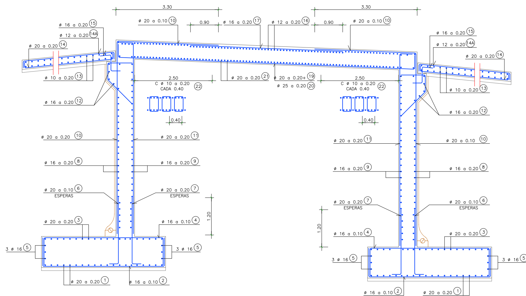
ARMAT SECCIÓ TRANSVERSAL A-A ESCALA 1:75
