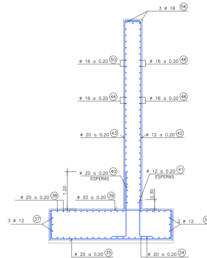
ARMAT SECCIÓ ALETA ESCALA 1:75
