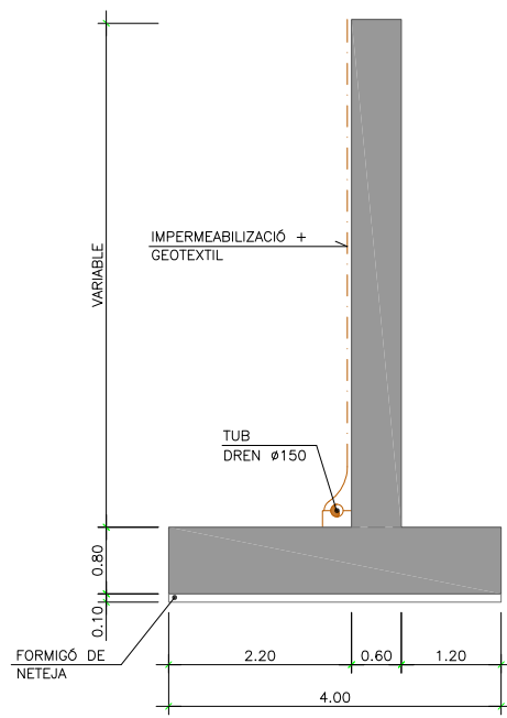
SECCIÓ ALETA ESCALA 1:100
