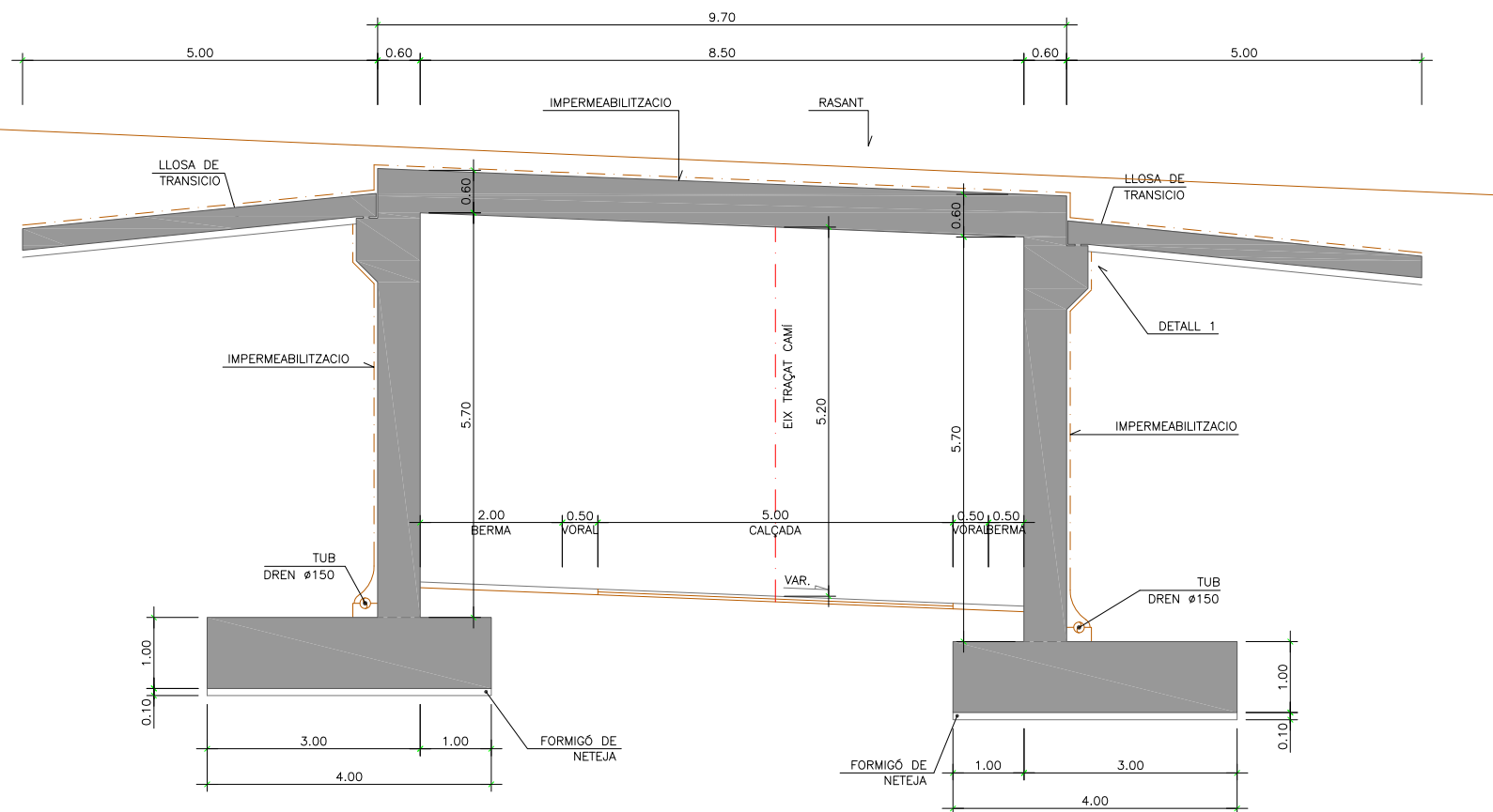
SECCIÓ TRANSVERSAL A-A ESCALA 1:100
