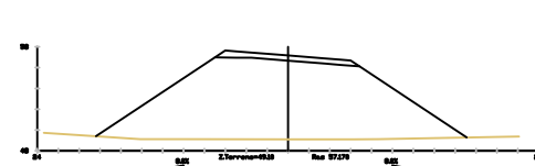
Pk=2+140 S. FINEC = 477 m. S. TORNAPLÉN = 3820 m.
