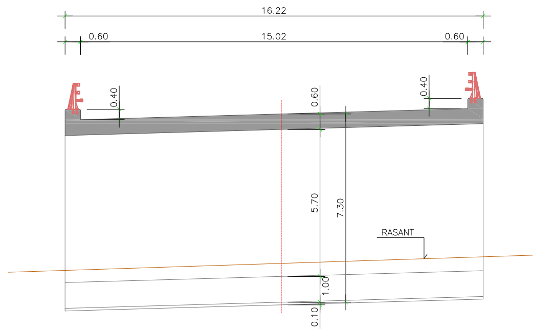
SECCIÓN LONGITUDINAL B-B ESCALA 1:150
