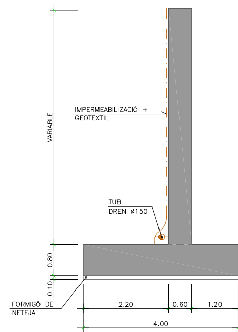
SECCIÓ ALETA ESCALA 1:100
