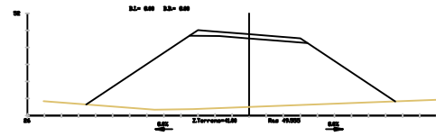
Pk=2+336.131 S. FINEC = 477 m. S. TORNAPLÉN = 3820 m.
