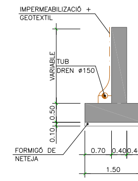
SECCIÓ ALETA ESCALA 1:100
