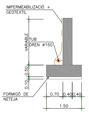
SECCIÓ ALETA ESCALA 1:100
