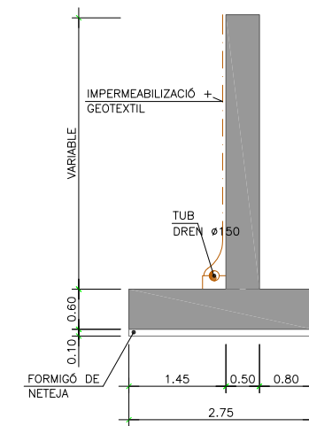
SECCIÓ ALETA ESCALA 1:100
