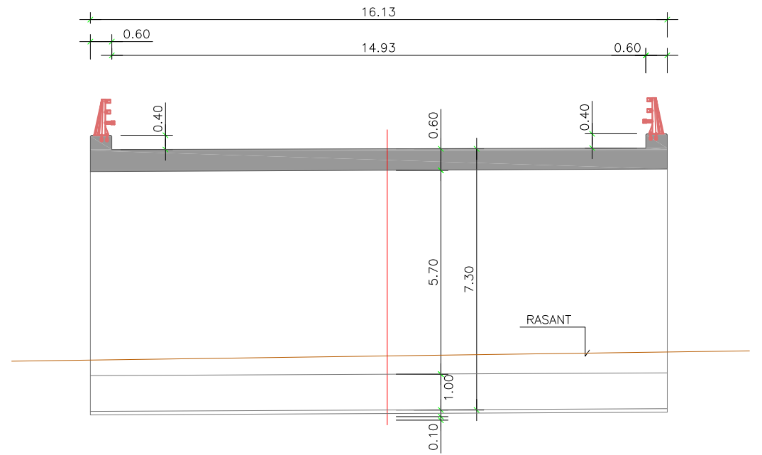
SECCIÓN LONGITUDINAL B-B ESCALA 1:150
