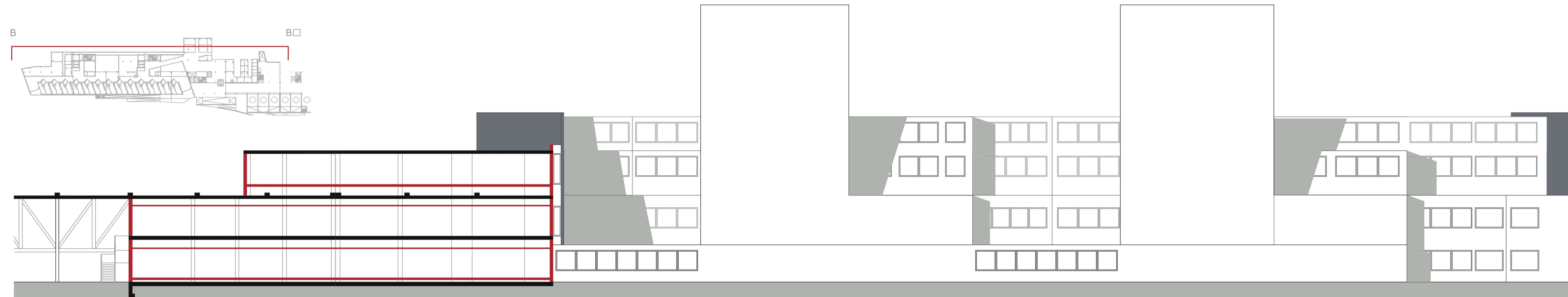
ALÇAT POSTERIOR B-B
