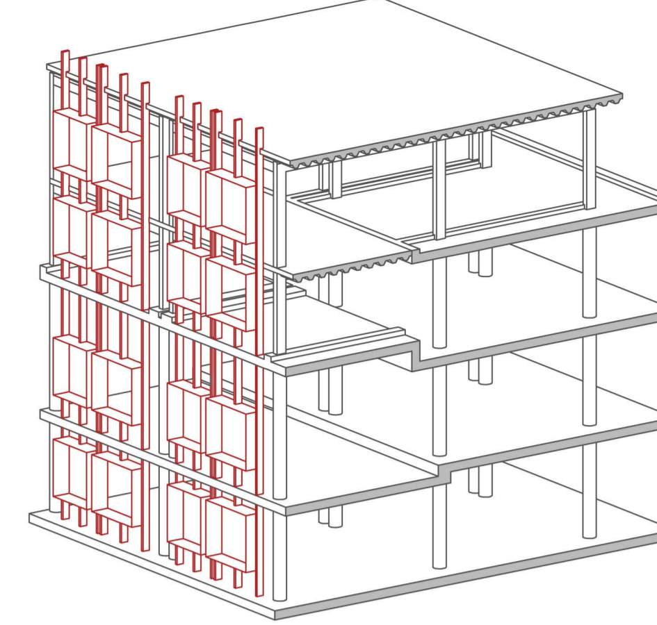
COL·LOCACIÓ DE FINESTRES I PROTECCIONS SOLARS
