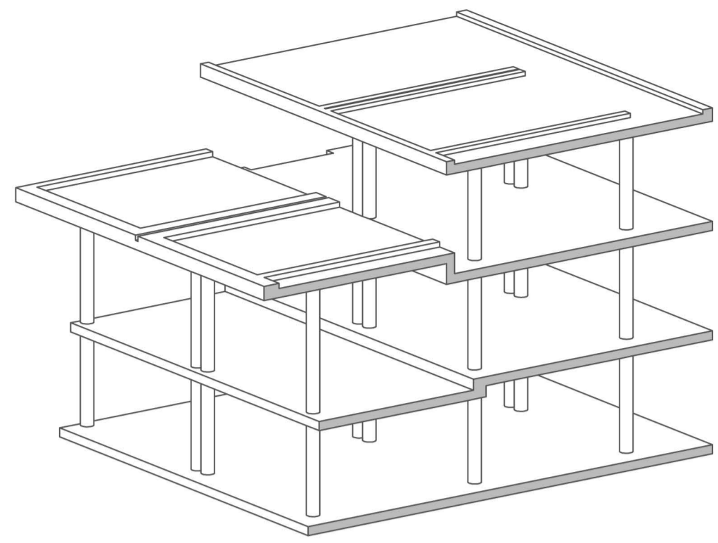
CONSTRUCCIÓ FULL DE FAÇANA INTERIOR I CREACIÓ DE PENDENT COBERTA
