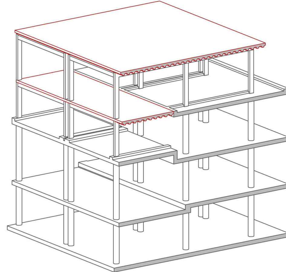
COL·LOCACIÓ D'APLACAT DE FAÇANA
