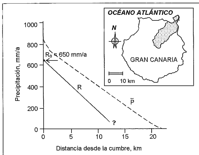
Figura 2. Evaluación de la recarga media a lo largo del sector nor-oriental (cuencas del Guinguada-Tenoya) de la isla de Gran Canaria con datos de pozos penetrantes, por lo que se ha considerado el efecto de acuífero en pendiente (Custodio, 2009)
