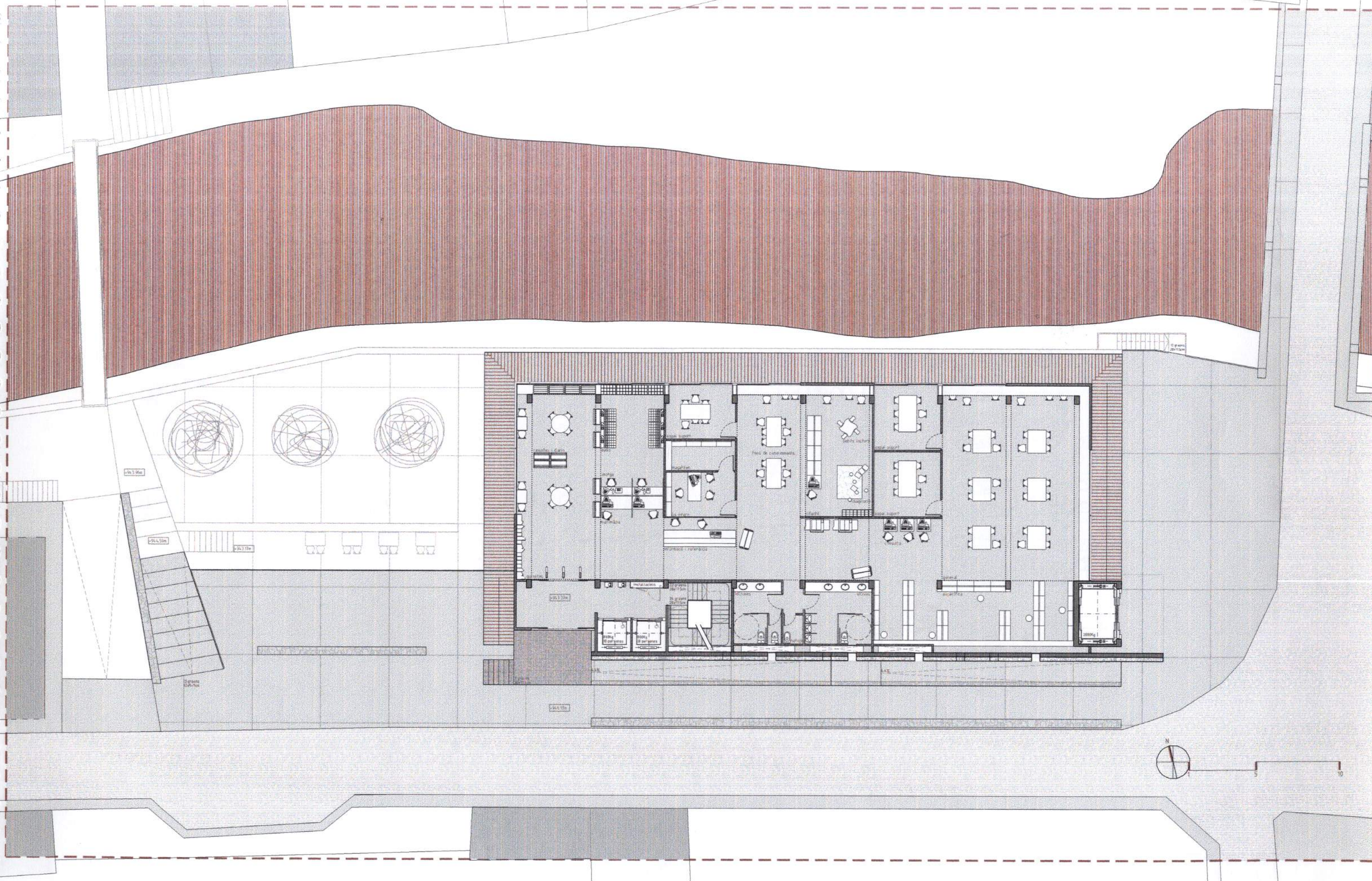
planta biblioteca [e: 1/100]
