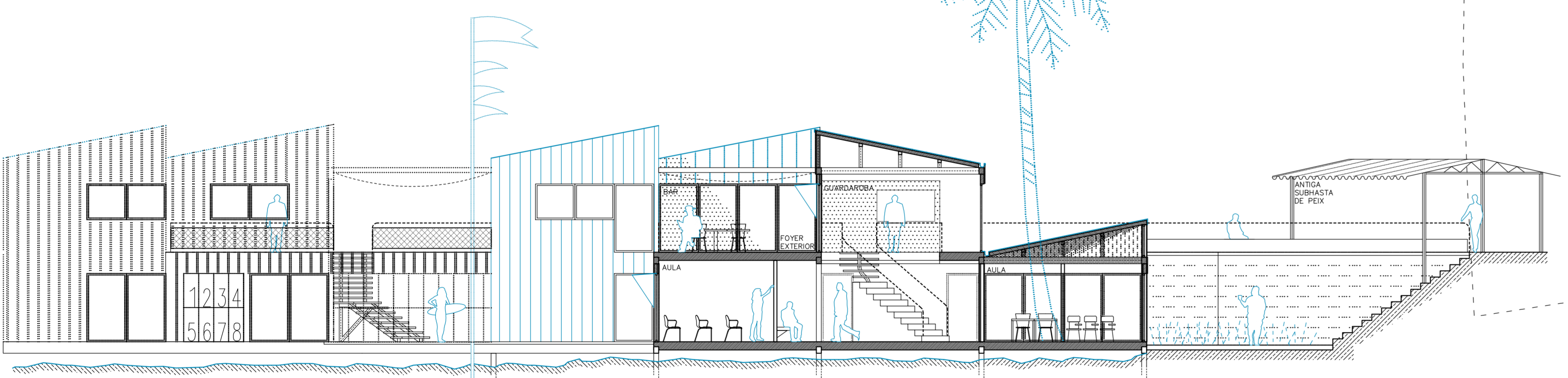
BB' SECCIÓ
