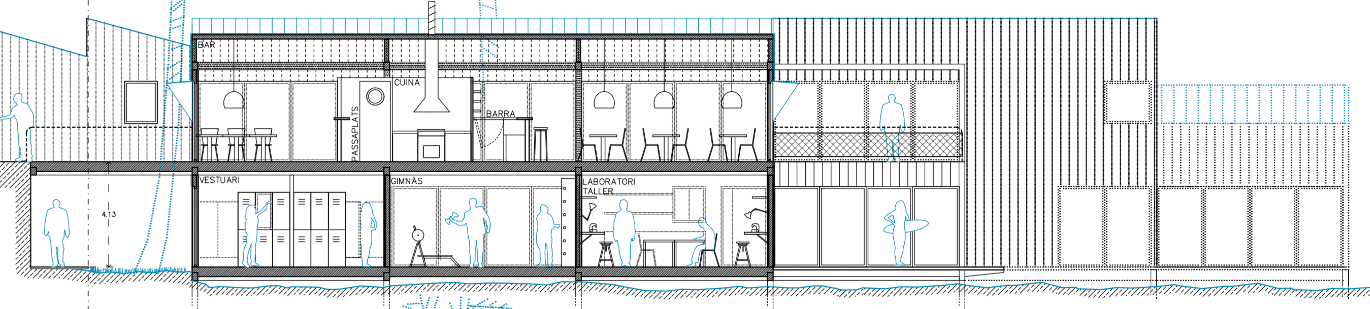
FF' SECCIÓ
