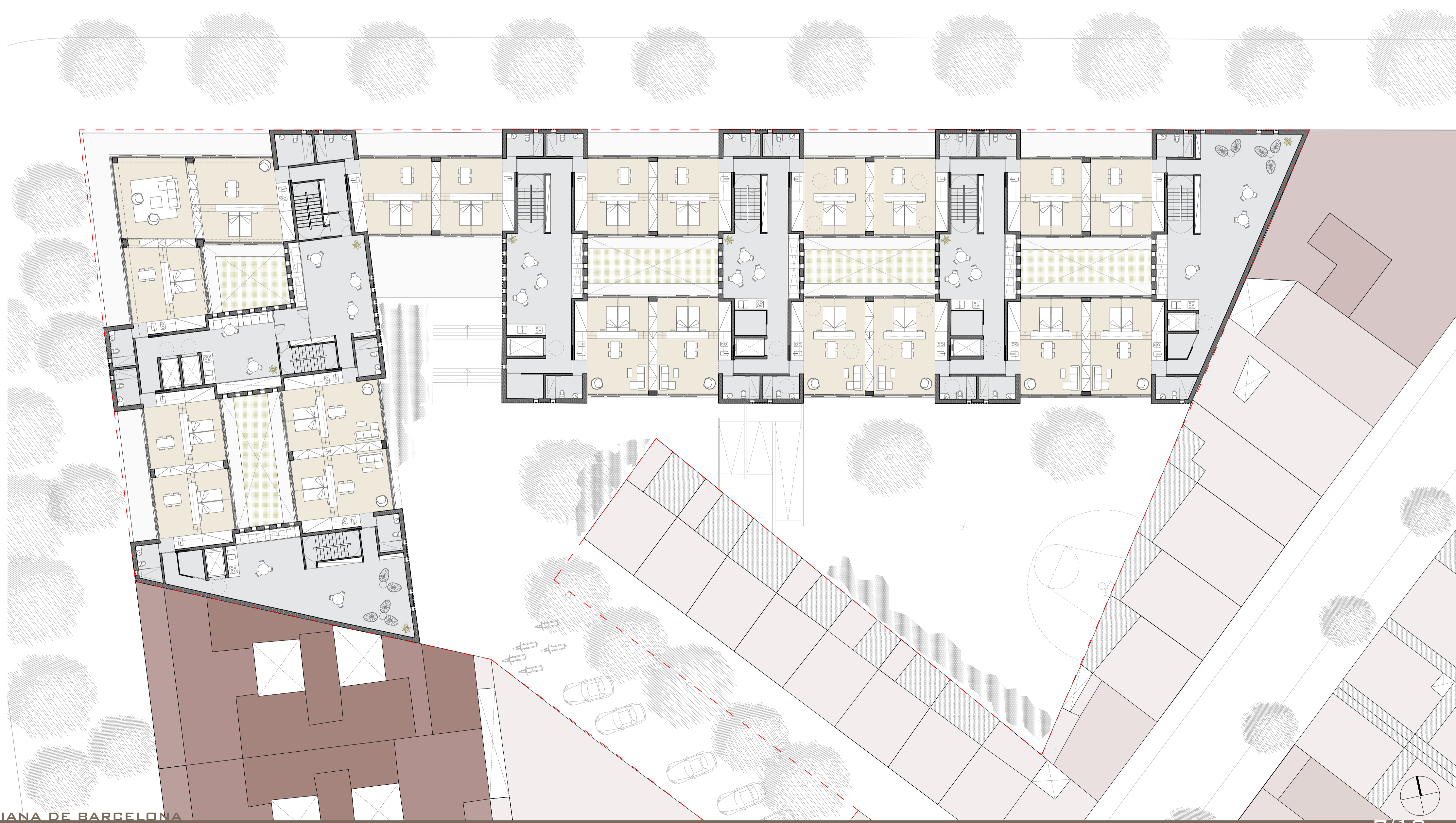
PLANTA TIPUS (P. SEGONA) ESCALA 1:200
