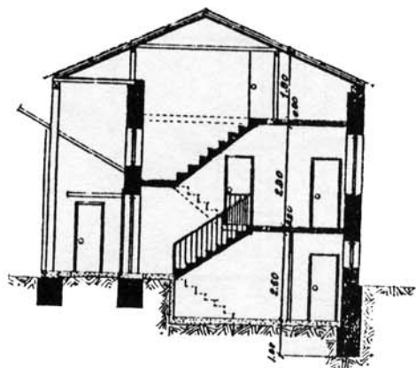
Sección X-X
