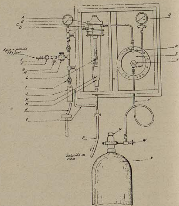
Aparato para la obtención de la solución de cloro Sistema Wallace and Tiernan Co.
