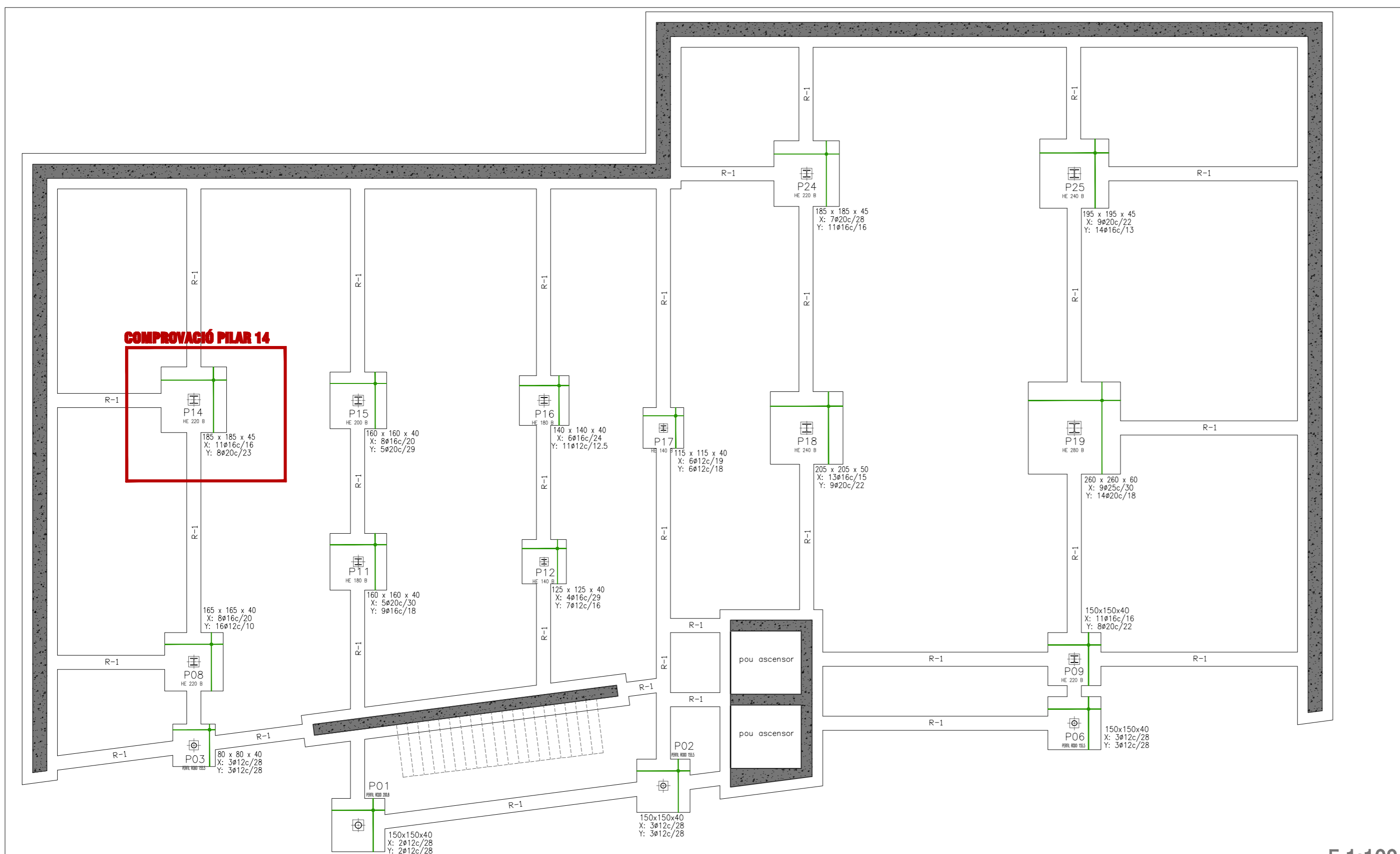
E 1:100
