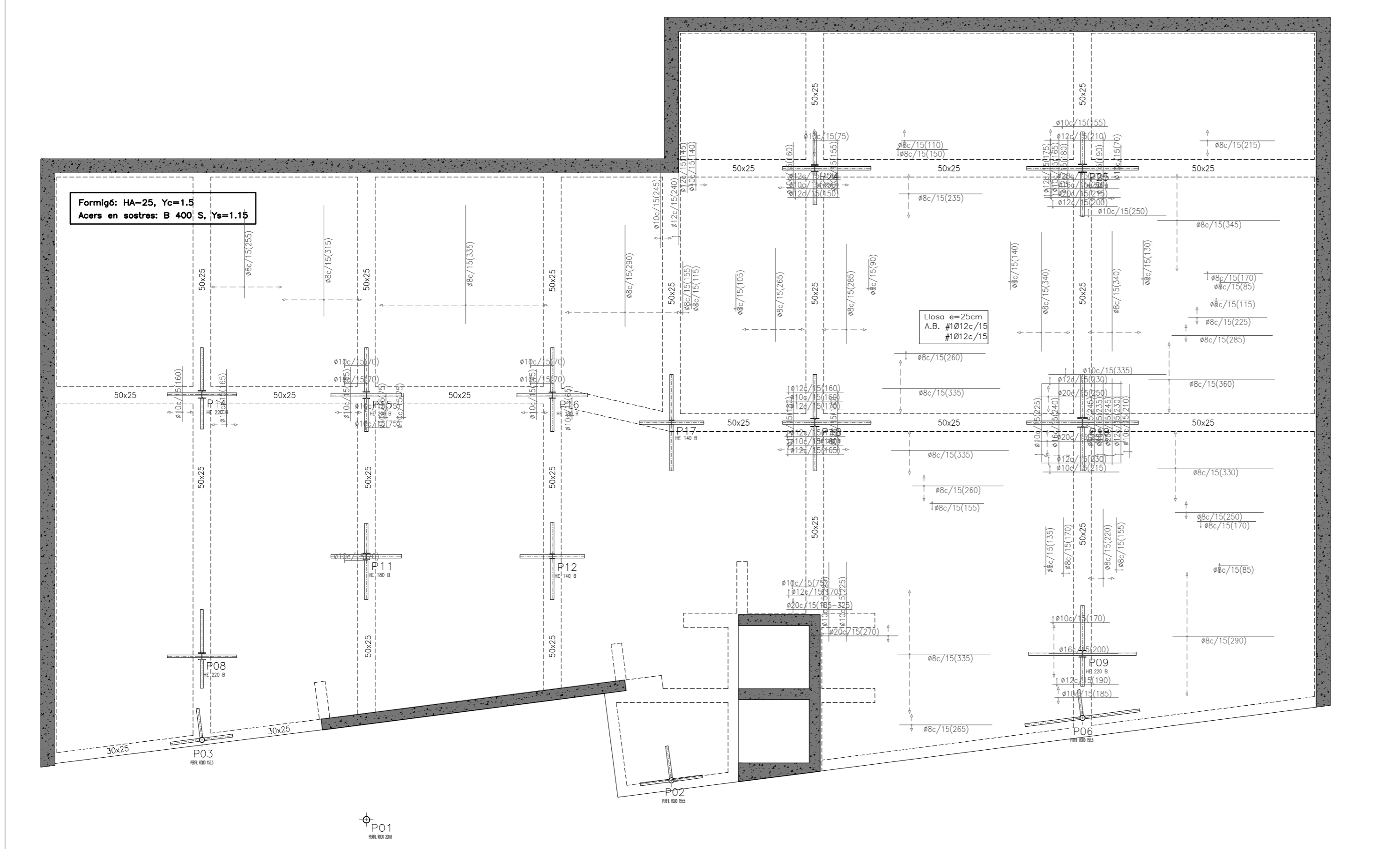
E 1:100
