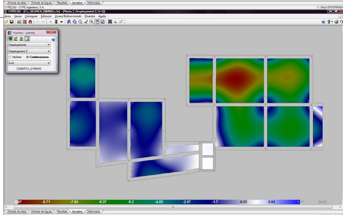
E 1:100
