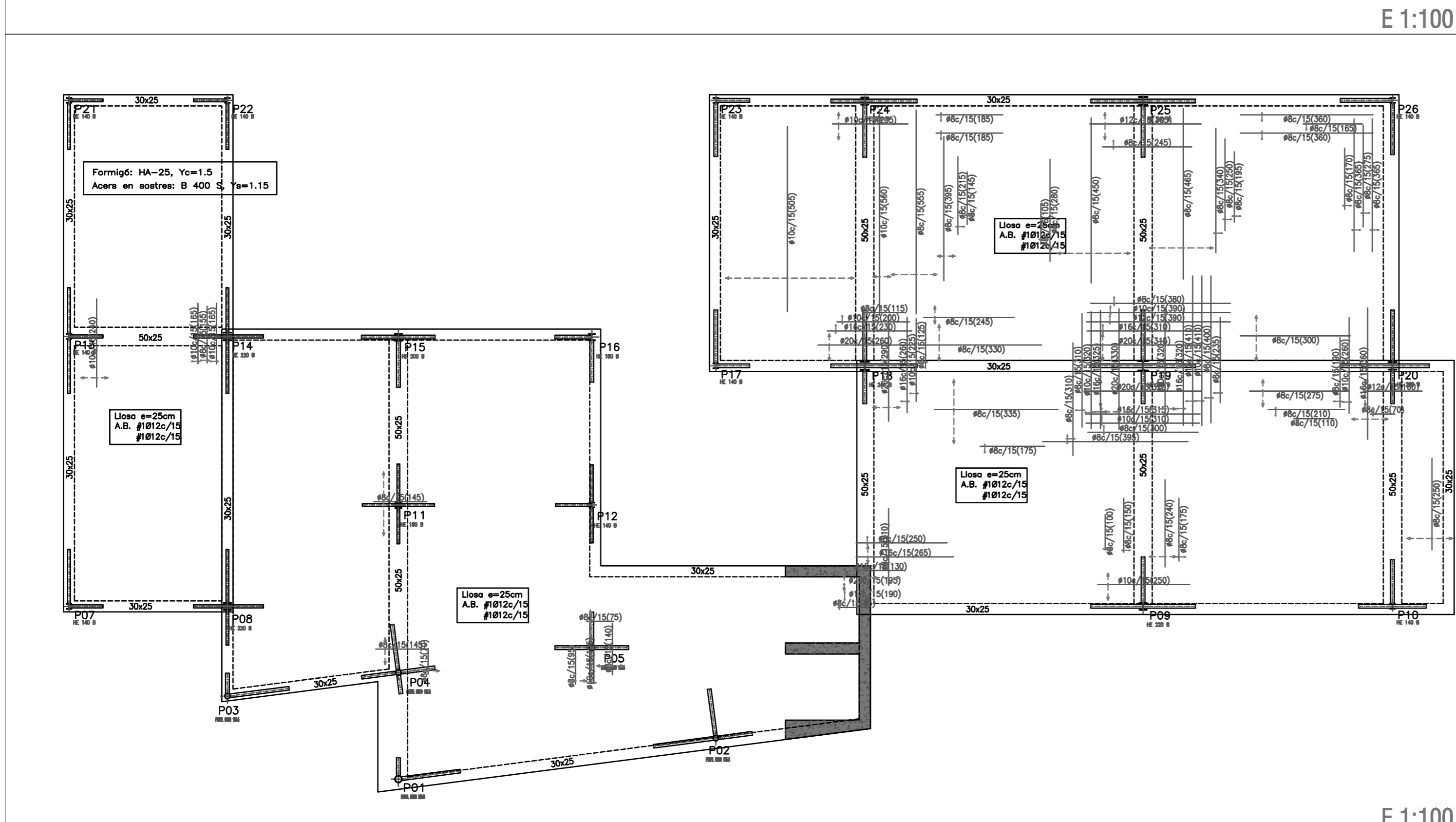
E 1:100
