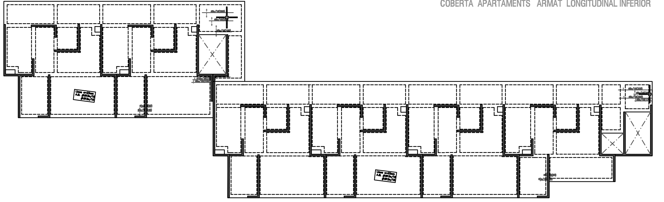
COBERTA APARTAMENTS ARMAT LONGITUDINAL SUPERIOR
