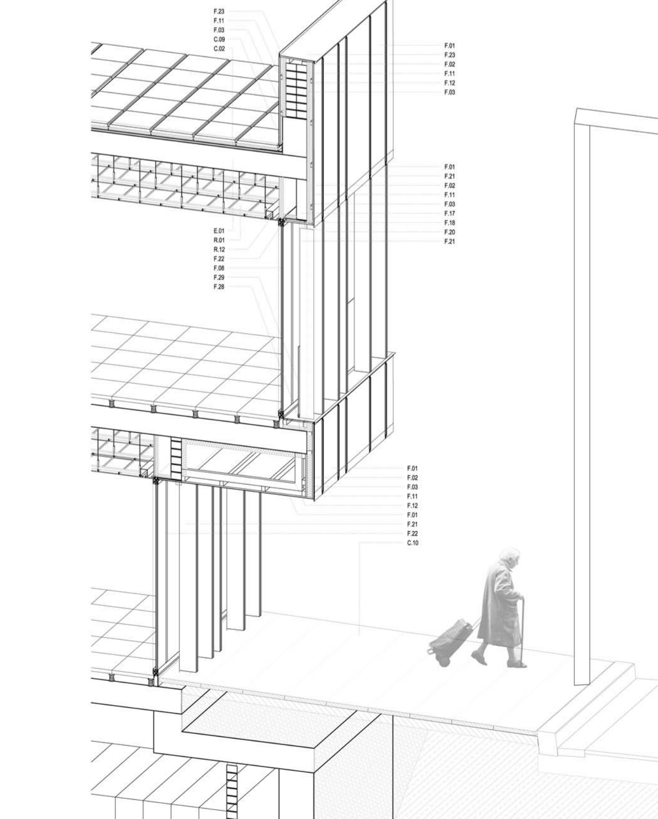
AXONOMETRIA SISTEMA CONSTRUCTIU
