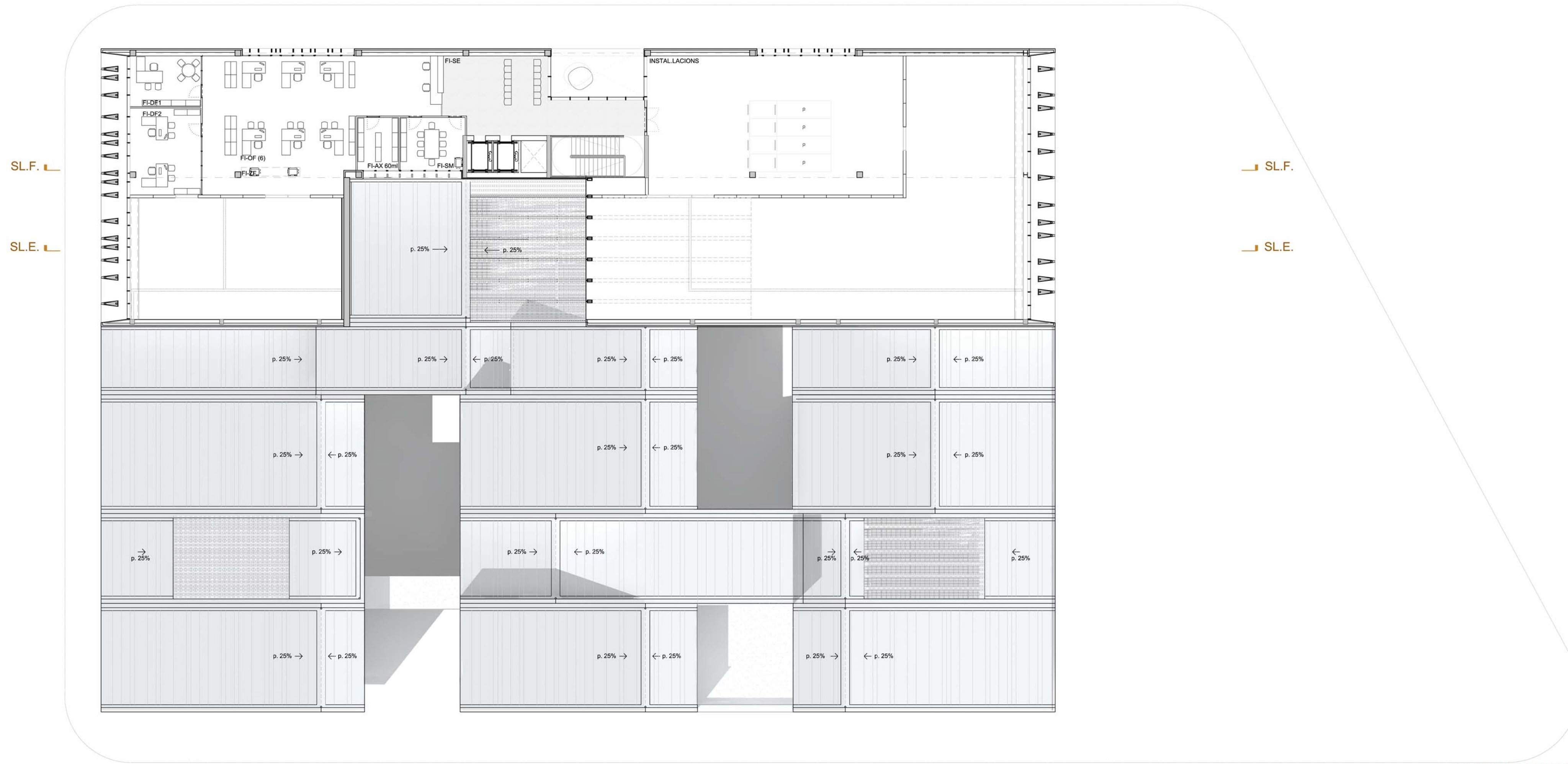
P.3. PLANTA TERCERA
