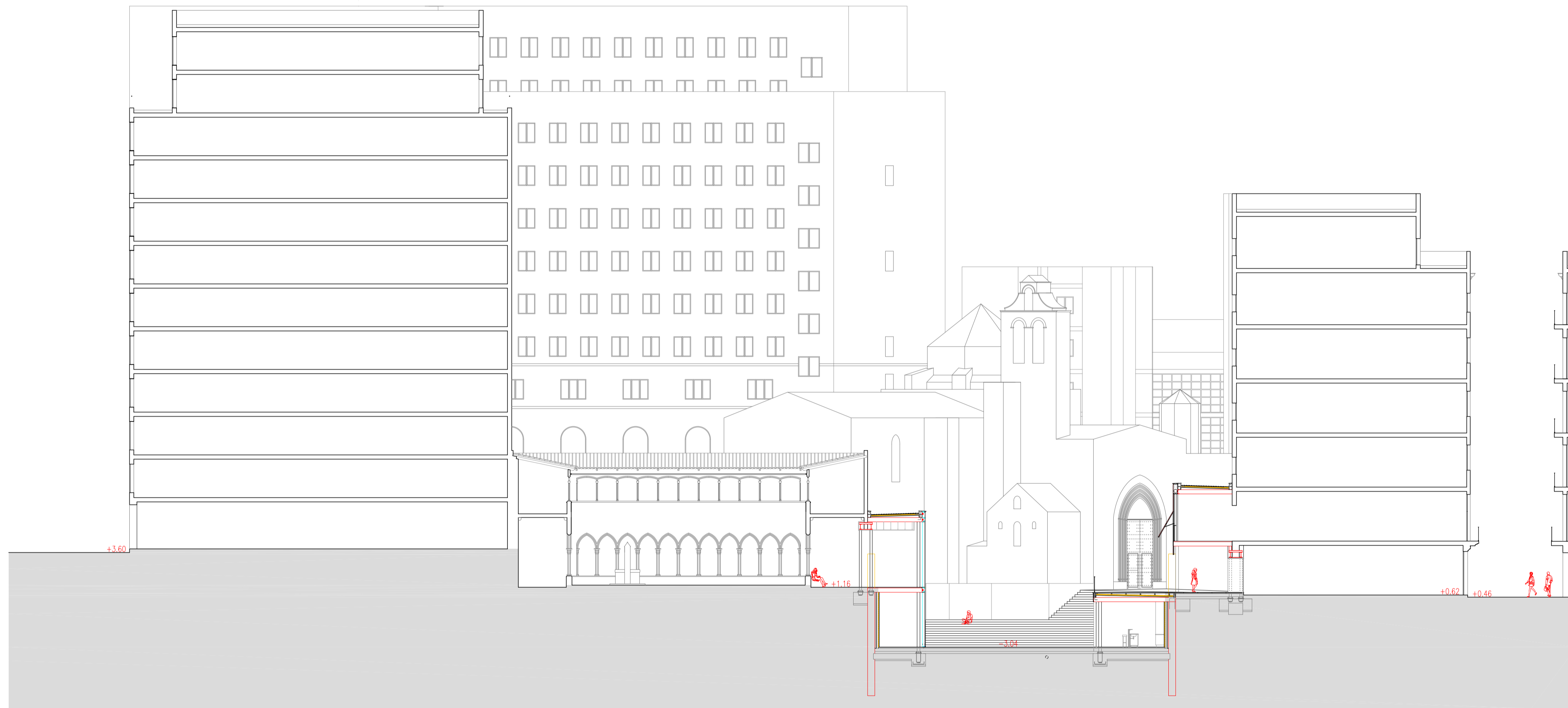
SECCIÓ TRANSVERSAL SS3
