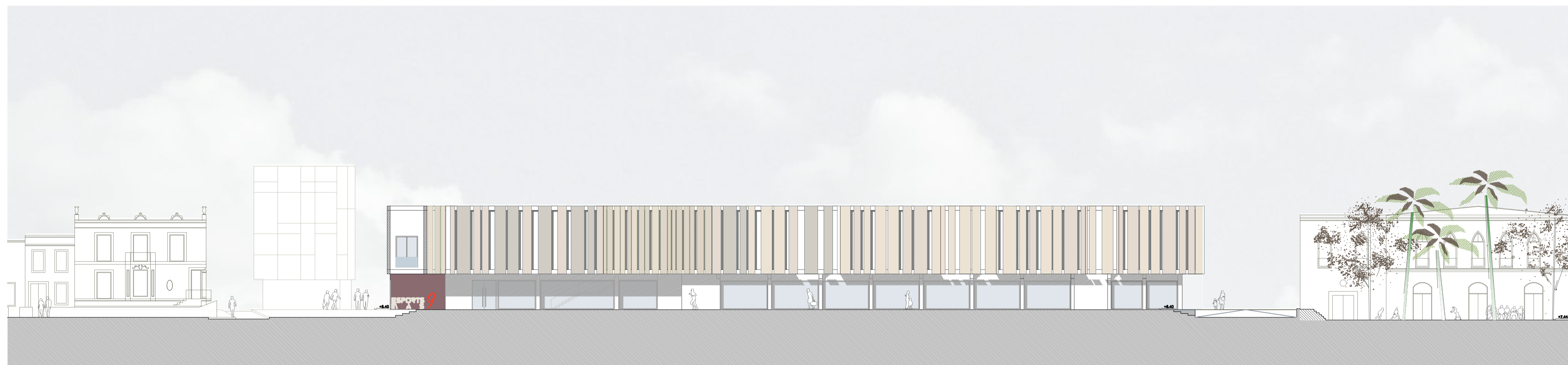
secció BB'
