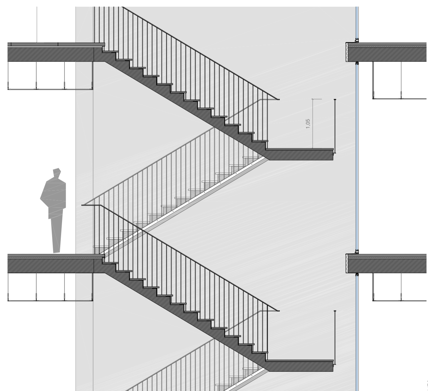
SECCIÓ GENERAL 1/50
