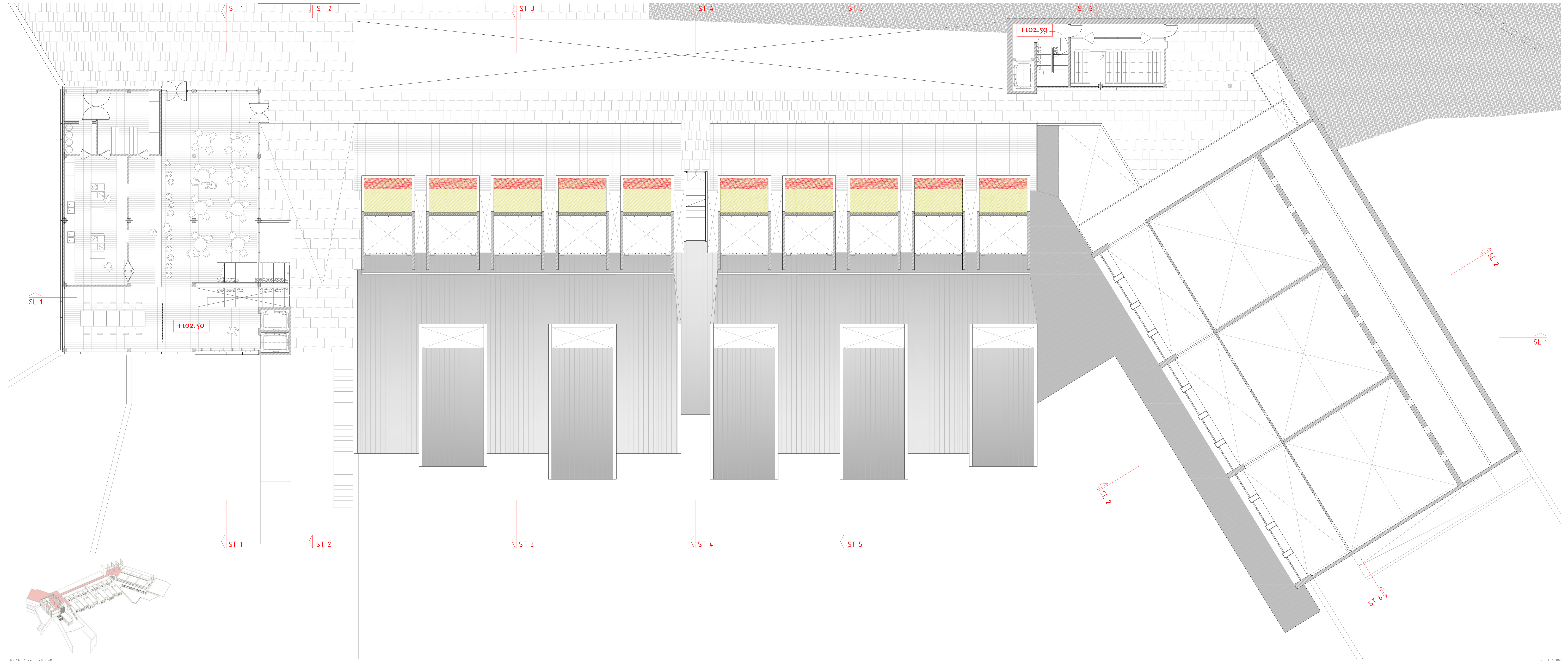
PLANTA cota +102.50
